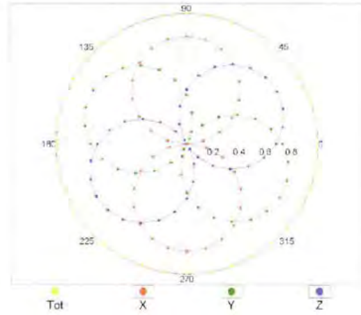
f=1800 MHz,R22
