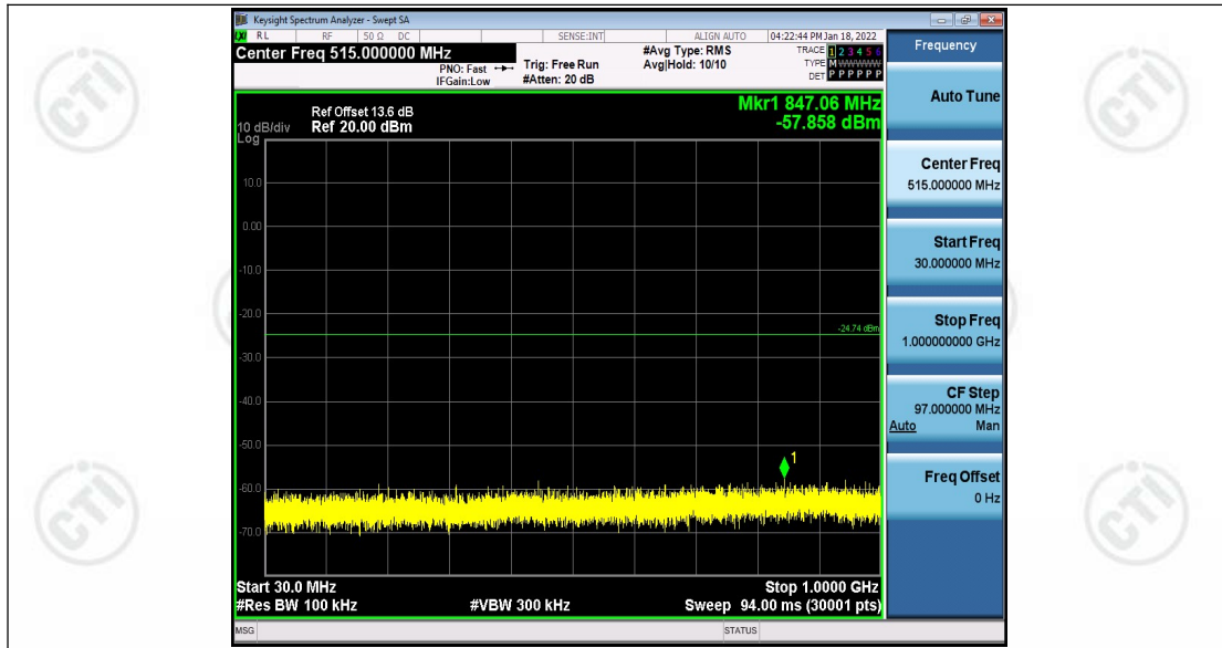
11G_Ant1_2412_30~1000
