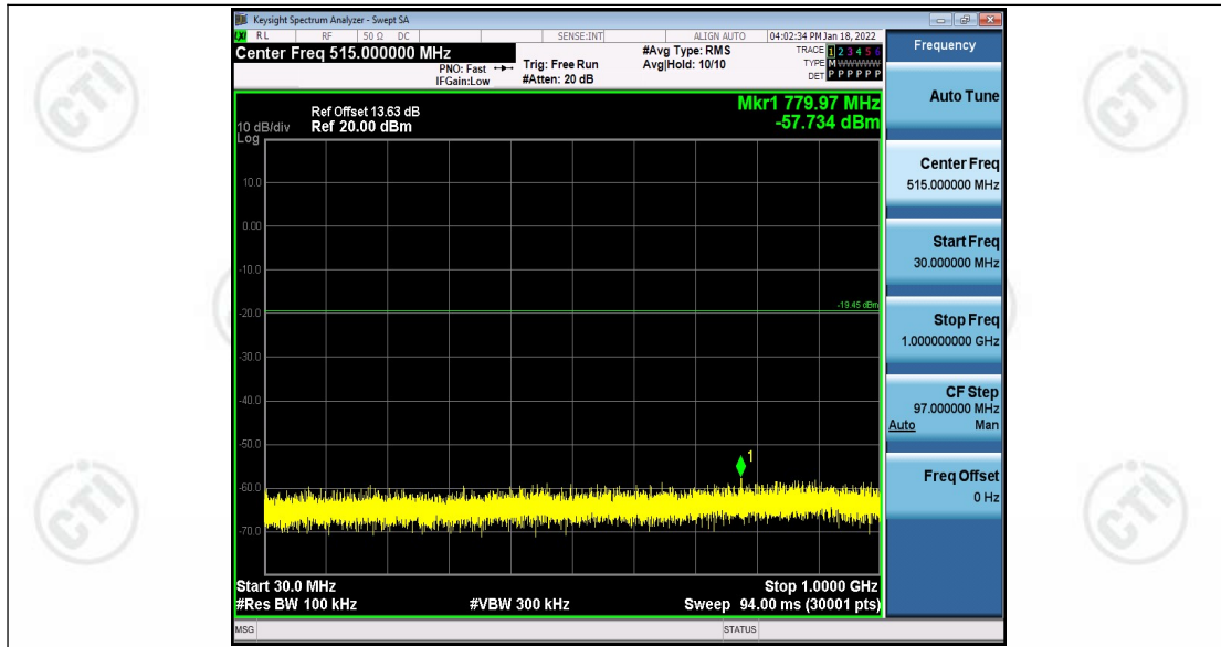
11B_Ant1_2437_30~1000
