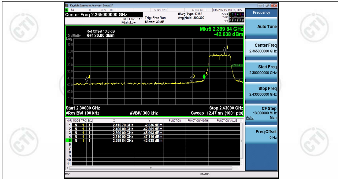
11G_Ant1_Low_2412
