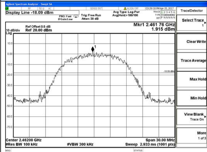
2447 – 2477 MHz
