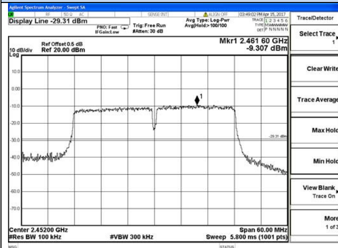
2422 – 2482 MHz
