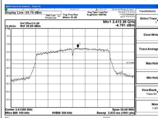
2397 – 2427 MHz
