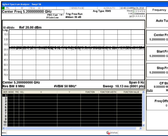
IEEE 802.11a
