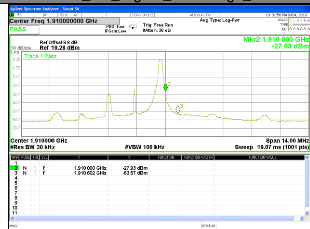
QPSK_3M_Higher_Band edge_1RB
