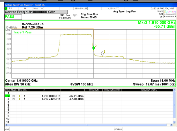
QPSK_3M_Higher_Band edge_FullRB
