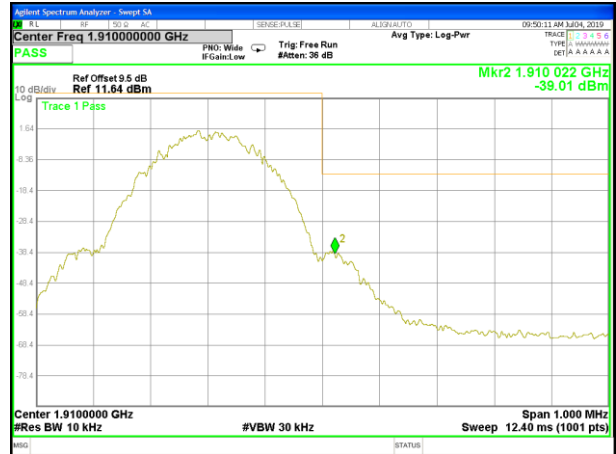
GPRS_1900_Higher_Band edge
