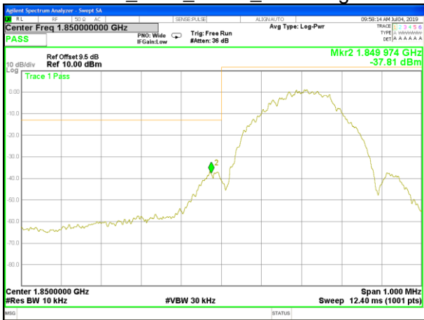
EGPRS_1900_Lower_Band edge
