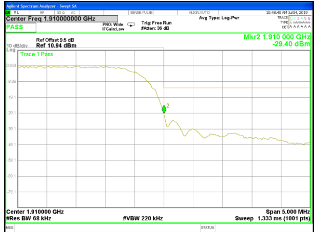
B2_WCDMA_Higher_Band edge
