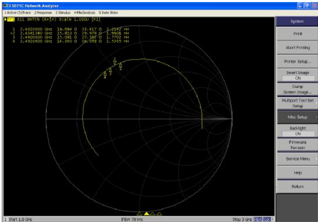
共轭匹配后
