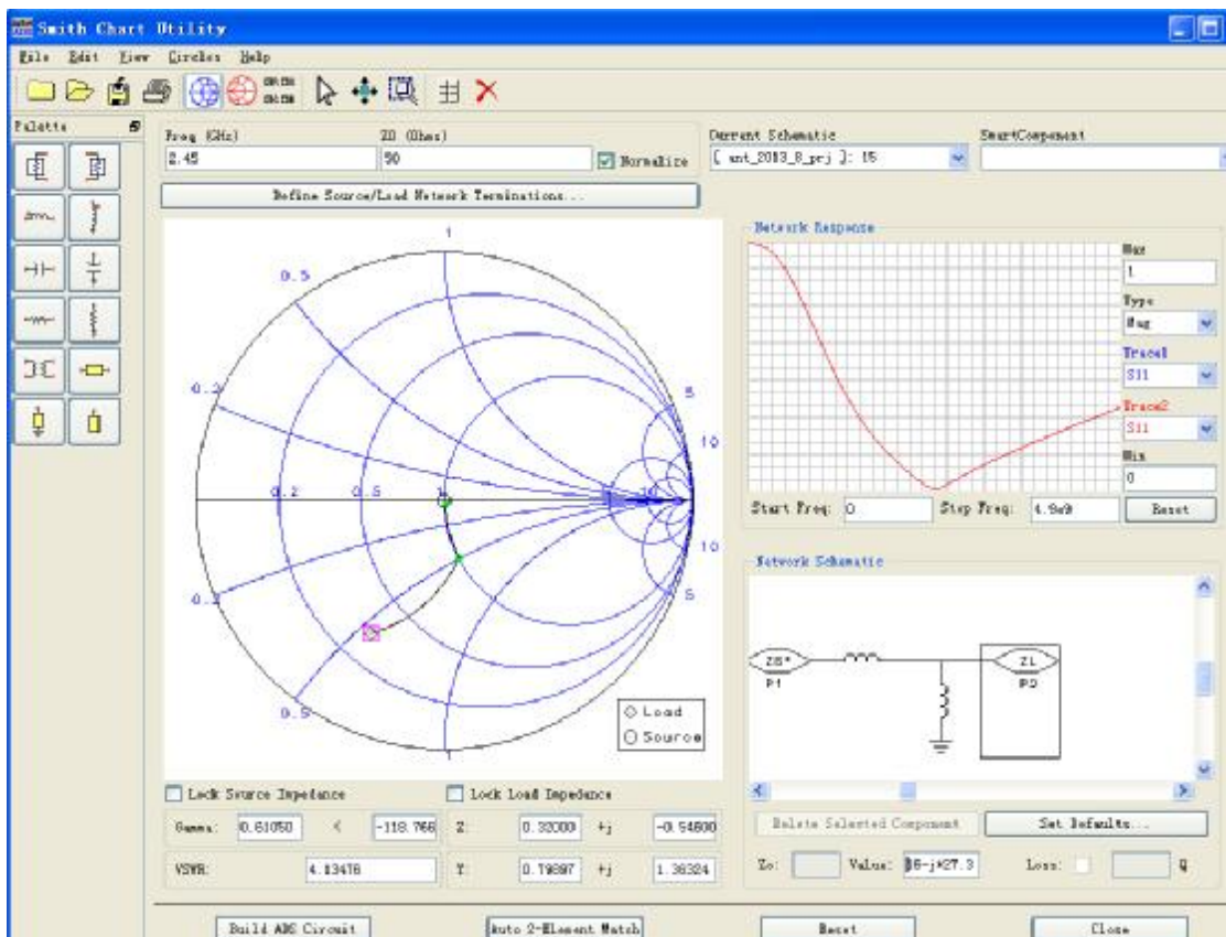
未进行匹配前的阻抗数据
