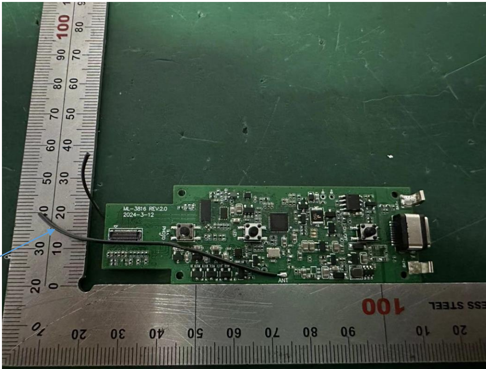
Internal photos M/N: Penguin CP1310F6
