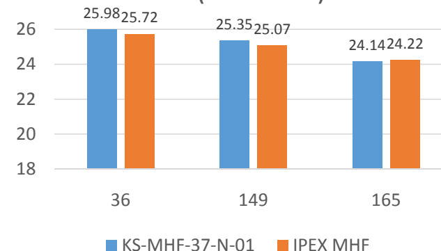
TRP (802.11ac)
