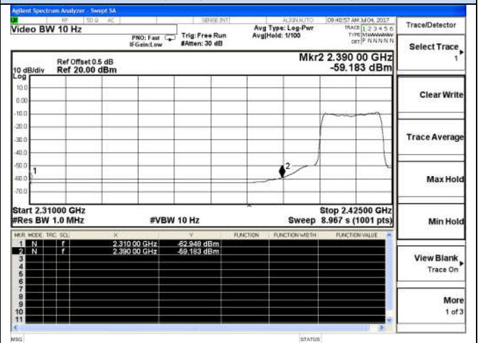
802.11n(HT20)-Low channel(Average)
