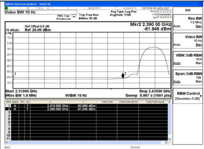
802.11b-Low channel(Average)
