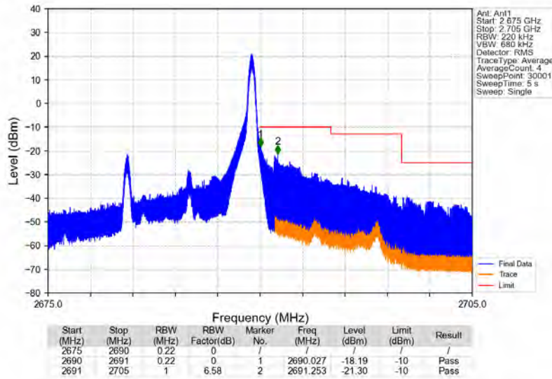
Band41_10MHz_64QAM_HCH_2685MHz_RB_1_49_NTNV
