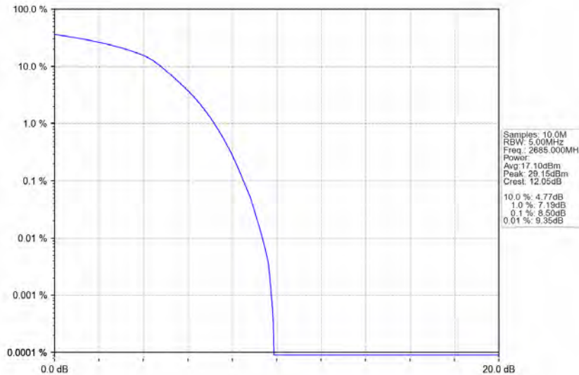
Band41_10MHz_16QAM_HCH_2685MHz_RB_50_0_NTNV
