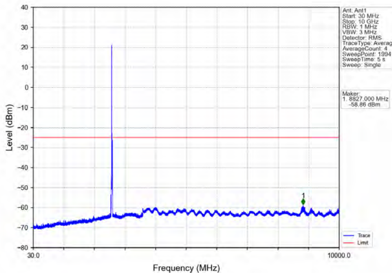
Band41_15MHz_QPSK_MCH_2593MHz_RB_1_0_NTNV
