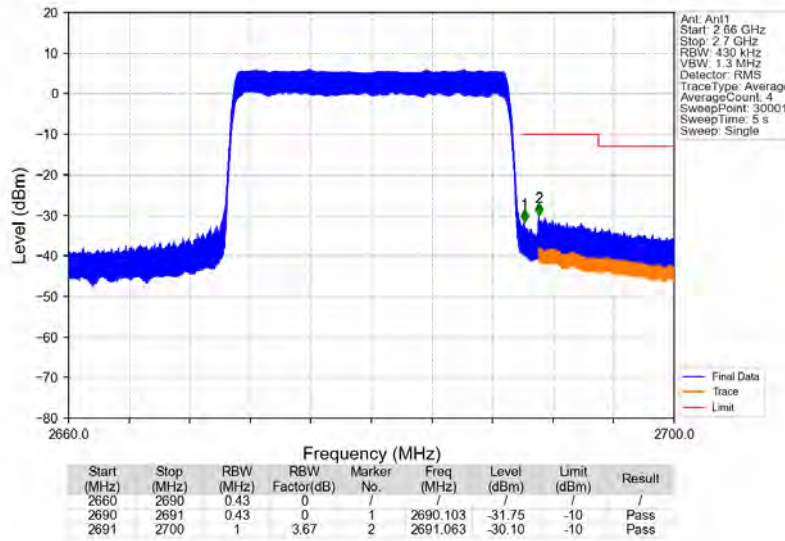
Band41_20MHz_QPSK_HCH_2680MHz_RB_100_0_NTNV
