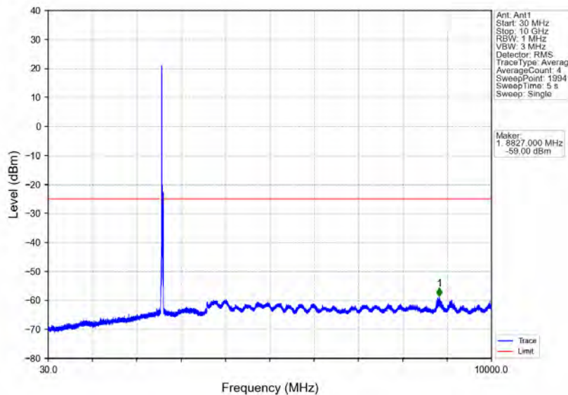
Band41_20MHz_QPSK_MCH_2593MHz_RB_1_0_NTNV
