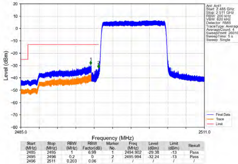
Band41_10MHz_QPSK_LCH_2501MHz_RB_50_0_NTNV
