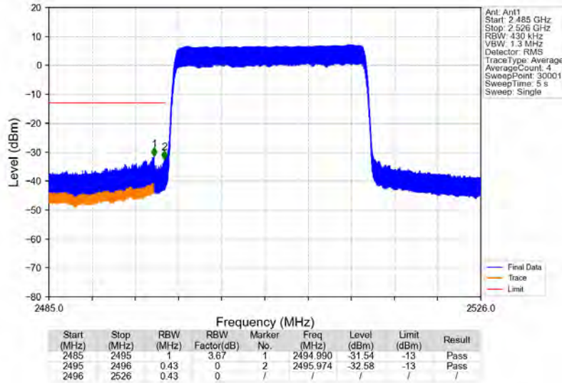
Band41_20MHz_QPSK_LCH_2506MHz_RB_100_0_NTNV
