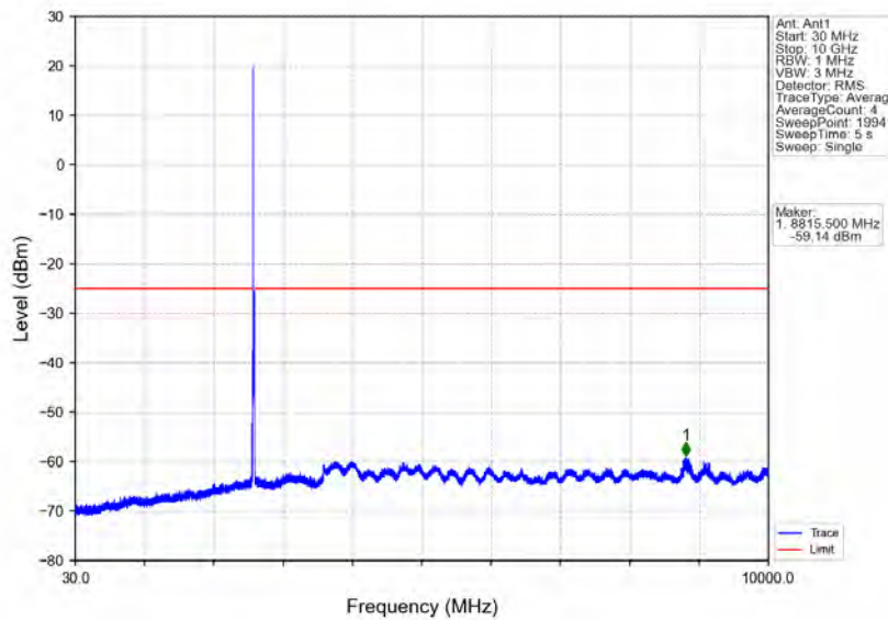
Band41_10MHz_QPSK_MCH_2593MHz_RB_1_0_NTNV
