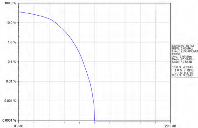
Band41_10MHz_16QAM_MCH_2593MHz_RB_50_0_NTNV
