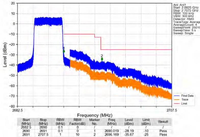
Band41_5MHz_QPSK_HCH_2687.5MHz_RB_25_0_NTNV
