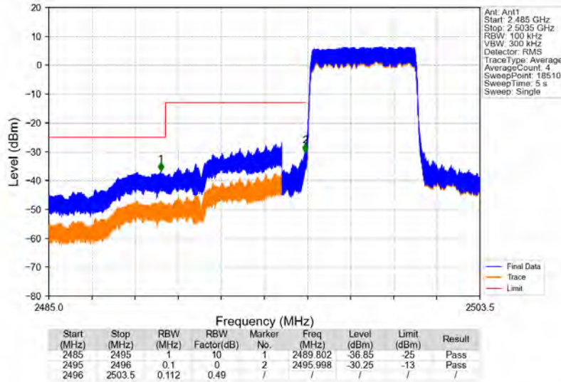
Band41_5MHz_QPSK_LCH_2498.5MHz_RB_25_0_NTNV
