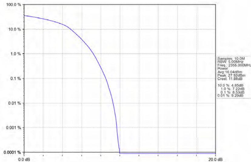
Band40b_10MHz_16QAM_LCH_2355MHz_RB_50_0_NTNV
