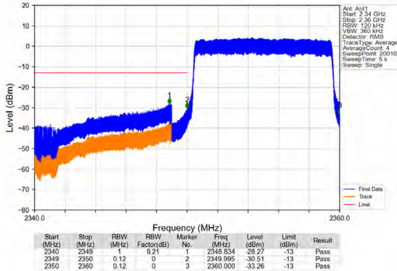
Band40b_10MHz_QPSK_LCH_2355MHz_RB_50_0_NTNV
