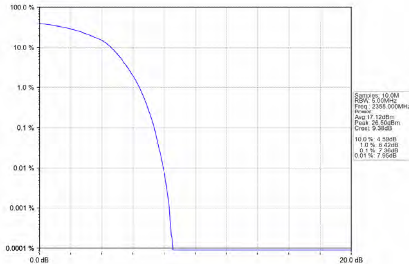
Band40b_10MHz_QPSK_HCH_2355MHz_RB_50_0_NTNV
