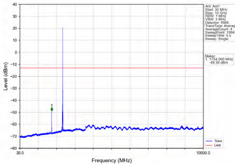
Band40b_5MHz_QPSK_MCH_2355MHz_RB_1_0_NTNV
