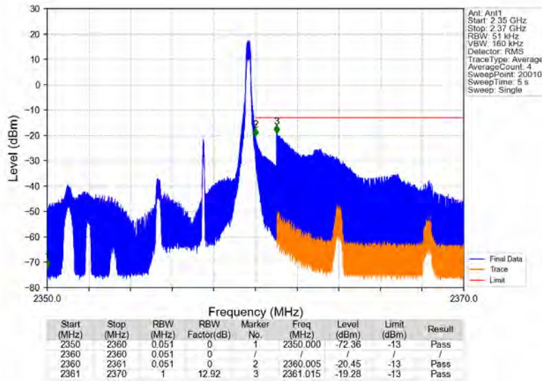
Band40b_5MHz_QPSK_HCH_2357.5MHz_RB_1_24_NTNV
