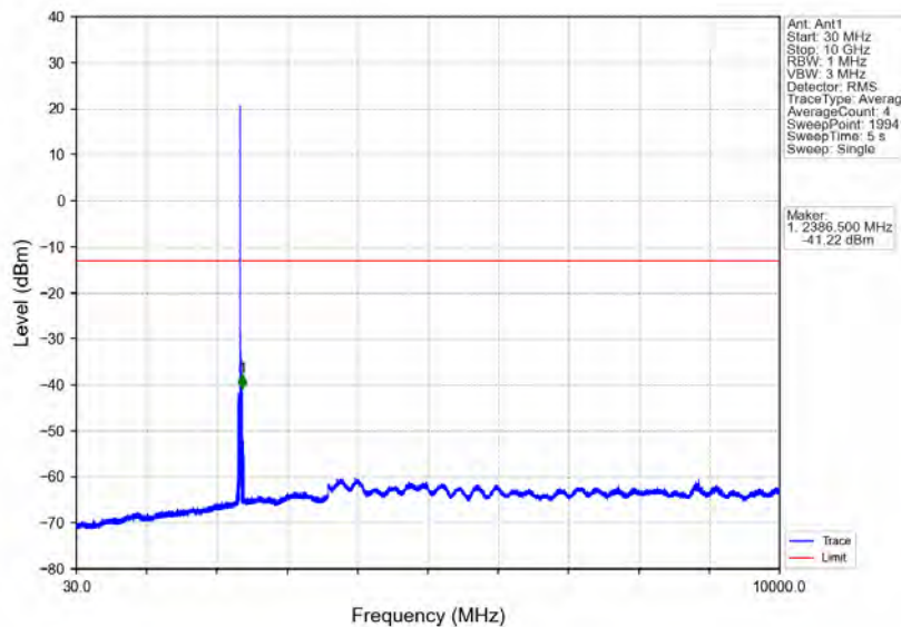
Band40b_10MHz_QPSK_MCH_2355MHz_RB_1_0_NTNV
