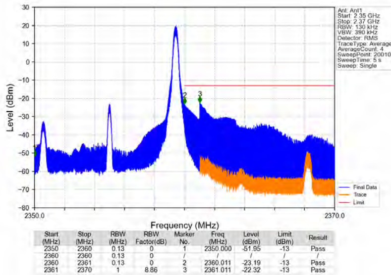
Band40b_10MHz_QPSK_HCH_2355MHz_RB_1_49_NTNV
