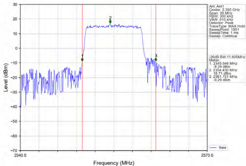
Band40b_10MHz_QPSK_LCH_2355MHz_RB_50_0_NTNV
