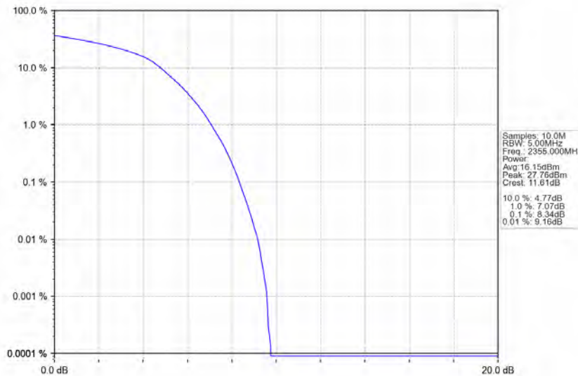
Band40b_10MHz_16QAM_MCH_2355MHz_RB_50_0_NTNV
