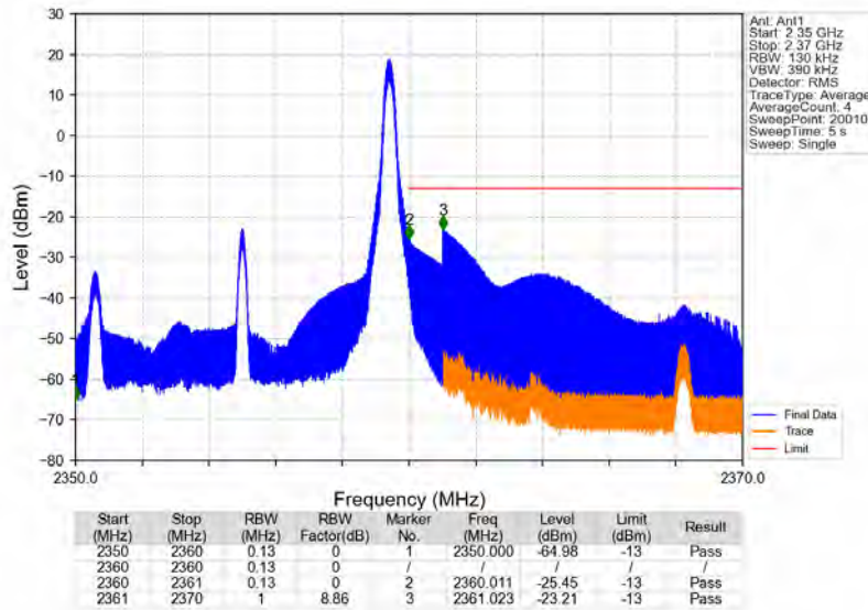
Band40b_10MHz_16QAM_HCH_2355MHz_RB_1_49_NTNV
