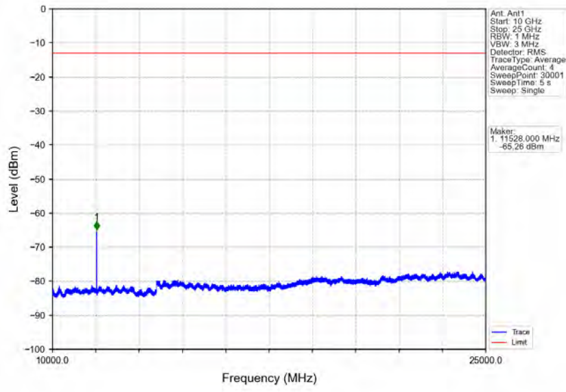
Band40a_10MHz_16QAM_MCH_2310MHz_RB_1_0_NTNV
