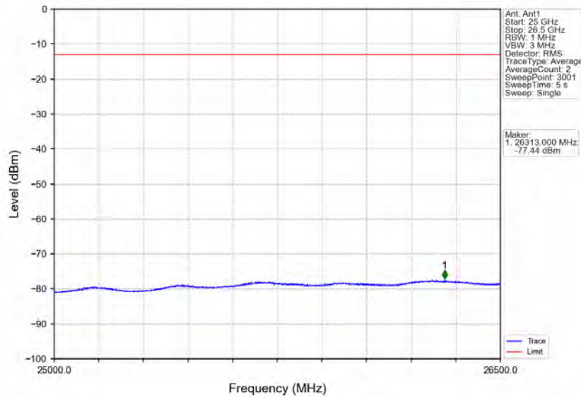
Band40a_5MHz_QPSK_HCH_2312.5MHz_RB_1_24_NTNV
