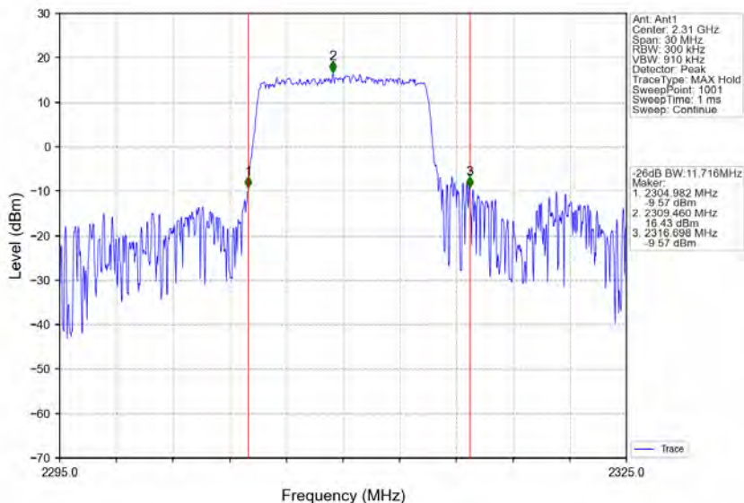
Band40a_10MHz_QPSK_HCH_2310MHz_RB_50_0_NTNV
