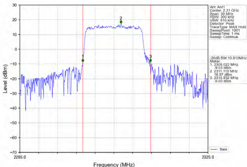
Band40a_10MHz_QPSK_HCH_2310MHz_RB_50_0_NTNV
