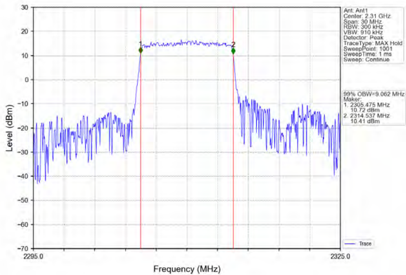
Band40a_10MHz_QPSK_HCH_2310MHz_RB_50_0_NTNV
