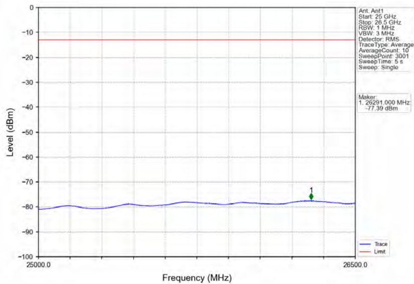
Band40a_10MHz_QPSK_LCH_2310MHz_RB_1_0_NTNV
