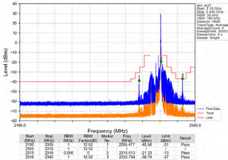
Band40a_5MHz_QPSK_HCH_2312.5MHz_RB_1_24_NTNV
