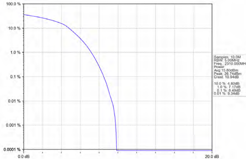
Band40a_10MHz_16QAM_LCH_2310MHz_RB_50_0_NTNV
