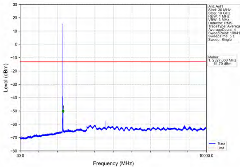
Band40a_5MHz_QPSK_MCH_2310MHz_RB_1_0_NTNV
