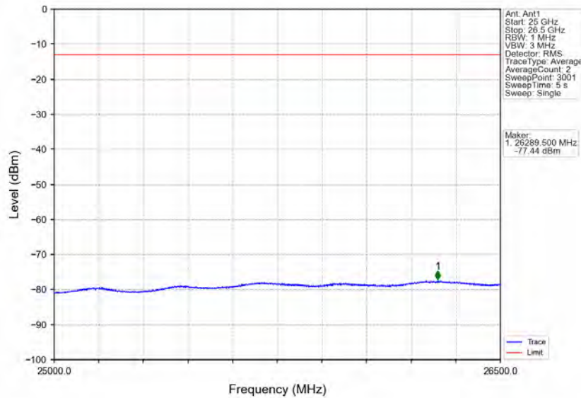
Band40a_10MHz_QPSK_MCH_2310MHz_RB_1_0_NTNV
