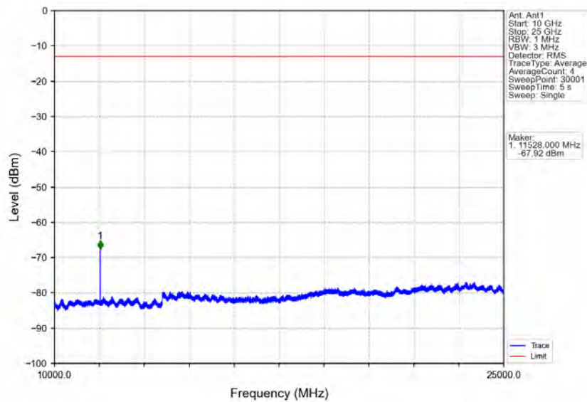
Band40a_10MHz_QPSK_HCH_2310MHz_RB_1_0_NTV
