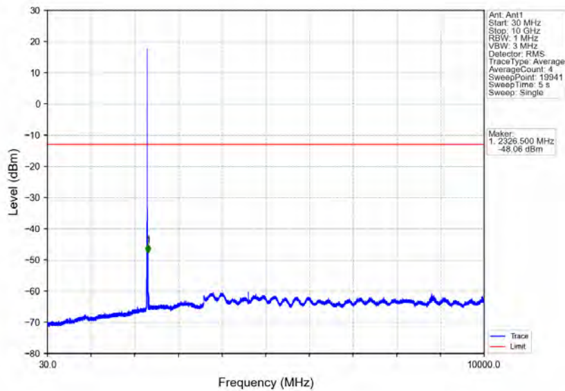
Band40a_5MHz_16QAM_MCH_2310MHz_RB_1_0_NTNV
