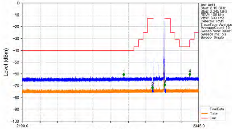
Band40a_10MHz_QPSK_HCH_2310MHz_RB_1_49_NTNV
