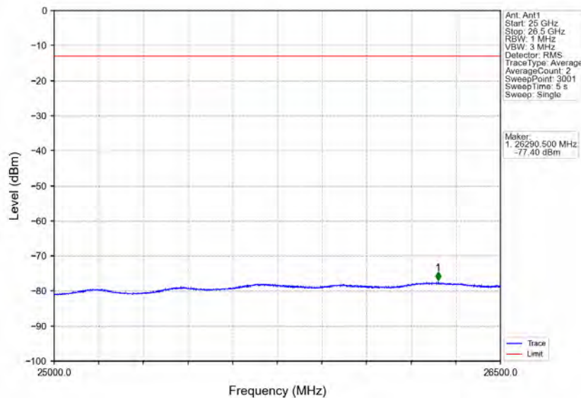
Band40a_5MHz_QPSK_LCH_2307.5MHz_RB_1_0_NTNV
