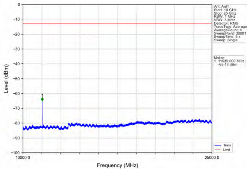
Band40a_5MHz_16QAM_MCH_2310MHz_RB_1_0_NTNV
