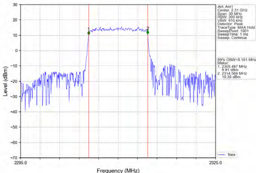
Band40a_10MHz_16QAM_MCH_2310MHz_RB_50_0_NTNV
