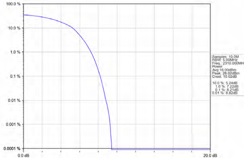
Band40a_10MHz_QPSK_HCH_2310MHz_RB_50_0_NTNV
