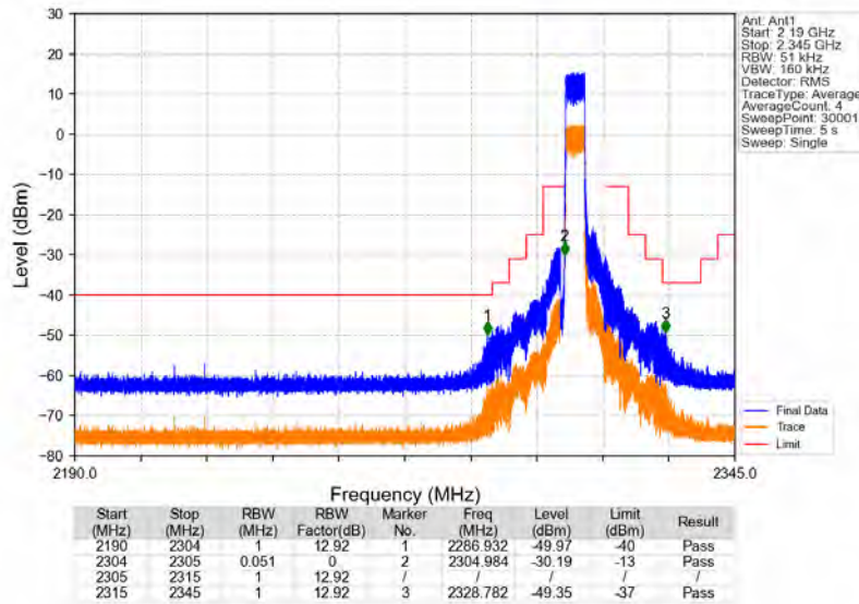
Band40a_5MHz_QPSK_MCH_2310MHz_RB_1_0_NTNV
