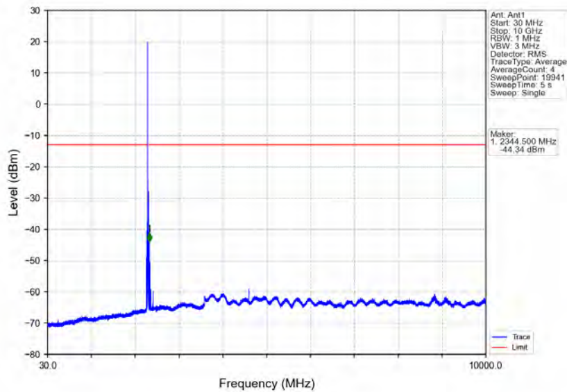
Band40a_10MHz_QPSK_HCH_2310MHz_RB_1_0_NTV
