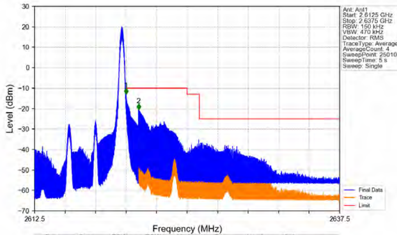
Band38_5MHz_QPSK_HCH_2617.5MHz_RB_1_24_NTNV
