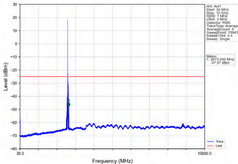
Band38_20MHz_16QAM_HCH_2610MHz_RB_1_0_NTV
