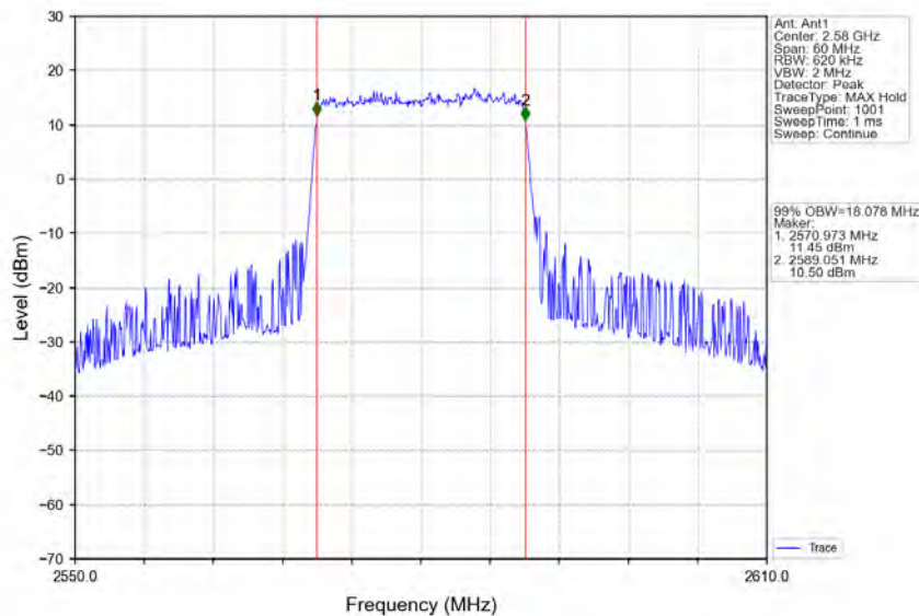
Band38_20MHz_64QAM_LCH_2580MHz_RB_100_0_NTNV
