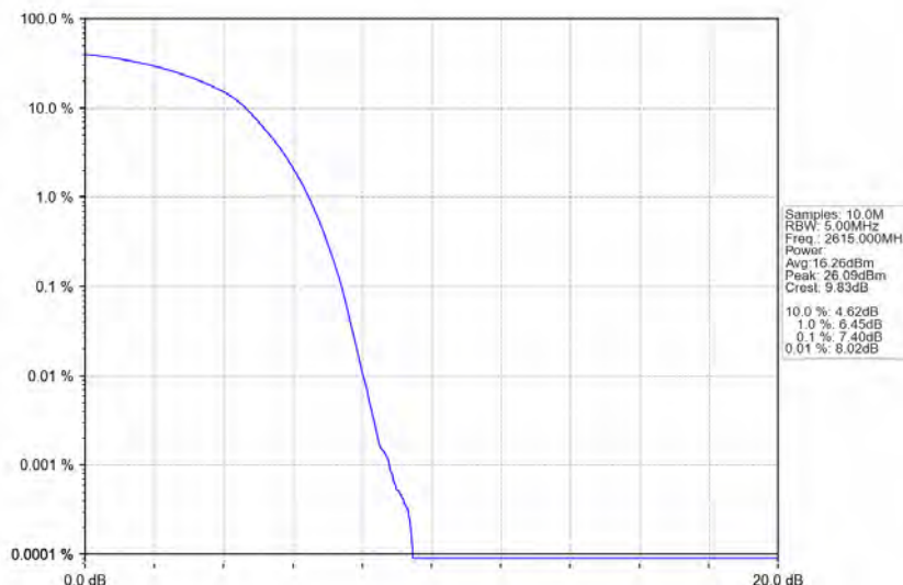
Band38_10MHz_QPSK_HCH_2615MHz_RB_50_0_NTNV
