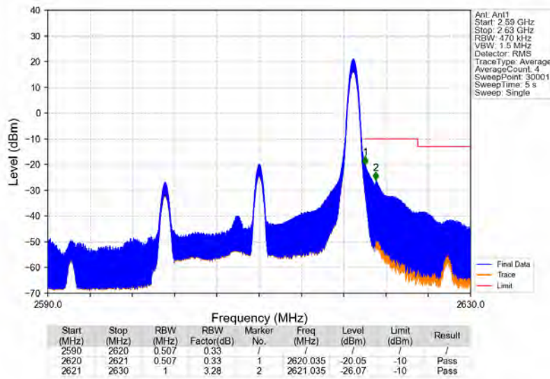
Band38_20MHz_QPSK_HCH_2610MHz_RB_1_99_NTNV
