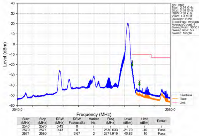
Band7_20MHz_64QAM_HCH_2560MHz_RB_1_99_NTNV
