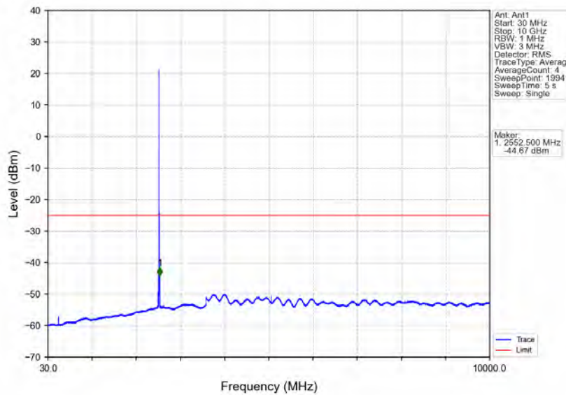
Band7_5MHz_QPSK_MCH_2535MHz_RB_1_0_NTNV
