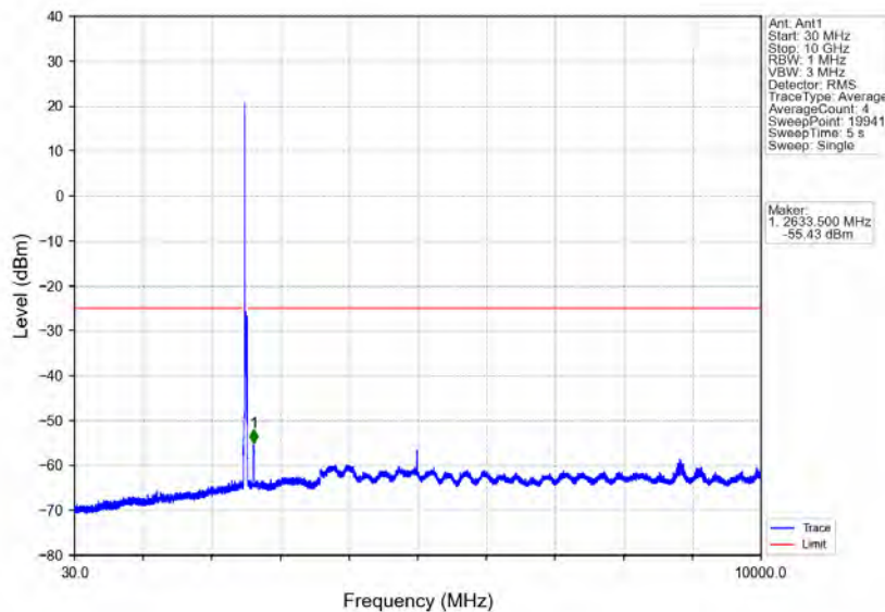
Band7_20MHz_64QAM_LCH_2510MHz_RB_1_0_NTNV
