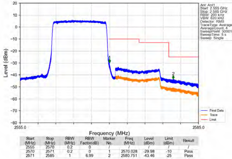
Band7_10MHz_QPSK_HCH_2565MHz_RB_50_0_NTNV
