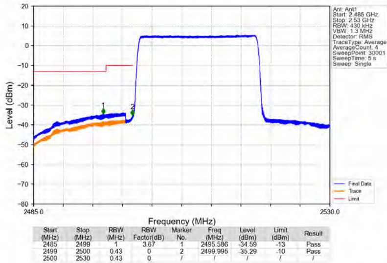
Band7_20MHz_64QAM_LCH_2510MHz_RB_100_0_NTNV
