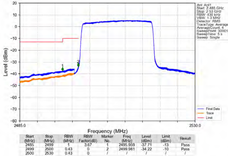
Band7_20MHz_QPSK_LCH_2510MHz_RB_100_0_NTNV
