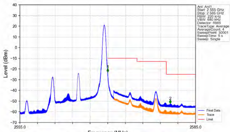
Band7_10MHz_QPSK_HCH_2565MHz_RB_1_49_NTNV
