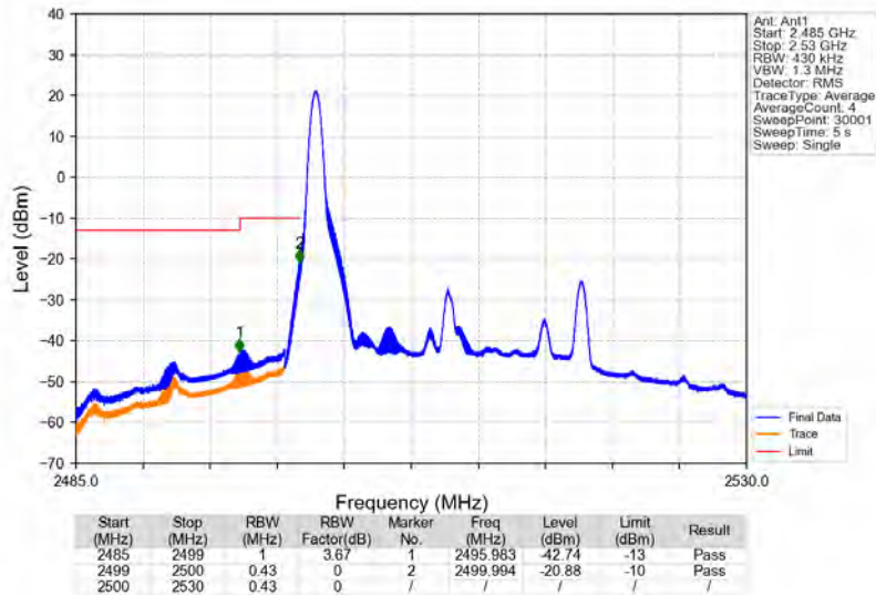
Band7_20MHz_64QAM_LCH_2510MHz_RB_1_0_NTNV
