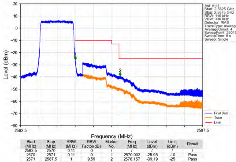
Band7_5MHz_QPSK_HCH_2567.5MHz_RB_25_0_NTNV
