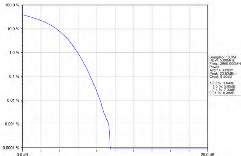
Band7_20MHz_16QAM_HCH_2560MHz_RB_100_0_NTNV
