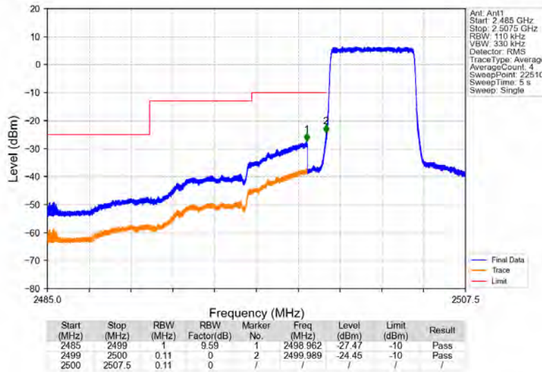
Band7_5MHz_QPSK_LCH_2502.5MHz_RB_25_0_NTNV
