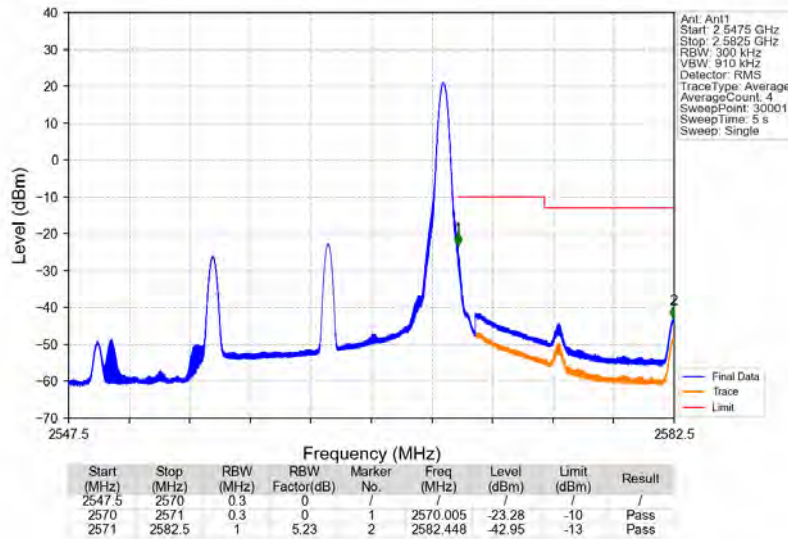
Band7_15MHz_QPSK_HCH_2562.5MHz_RB_1_74_NTNV
