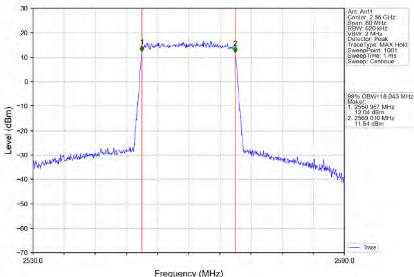
Band7_20MHz_64QAM_HCH_2560MHz_RB_100_0_NTNV
