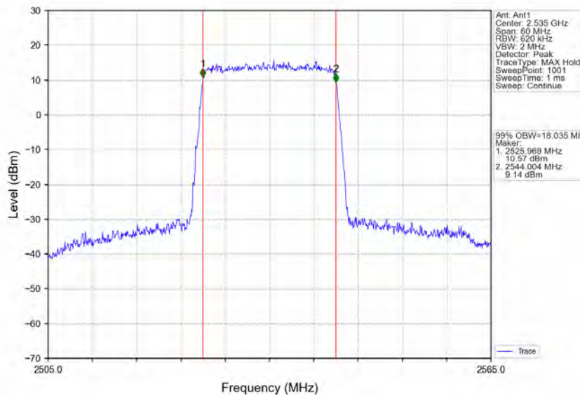
Band7_20MHz_16QAM_MCH_2535MHz_RB_100_0_NTNV
