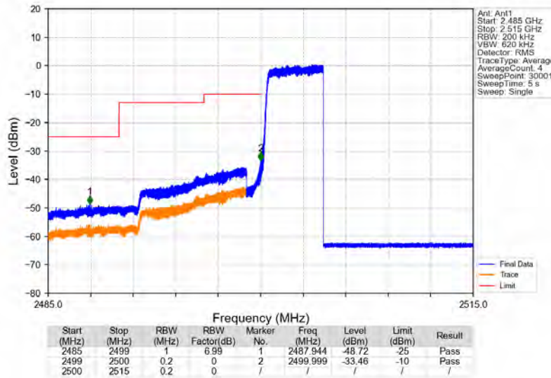
Band7_10MHz_QPSK_LCH_2505MHz_RB_50_0_NTNV
