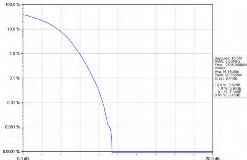
Band7_20MHz_16QAM_MCH_2535MHz_RB_100_0_NTNV
