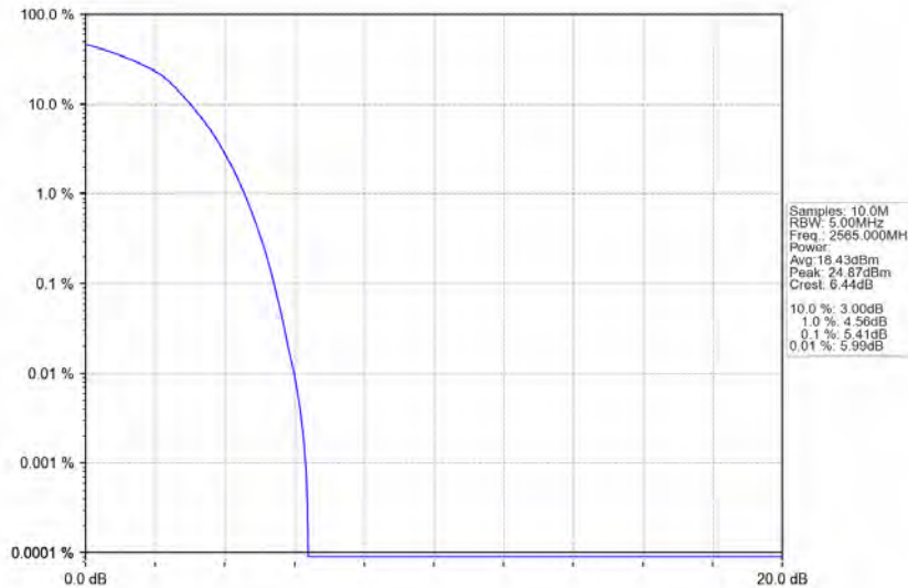
Band7_10MHz_QPSK_HCH_2565MHz_RB_50_0_NTNV
