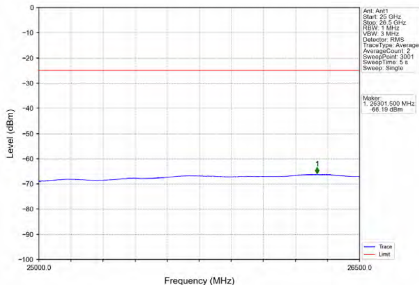
Band7_10MHz_QPSK_HCH_2565MHz_RB_1_49_NTNV
