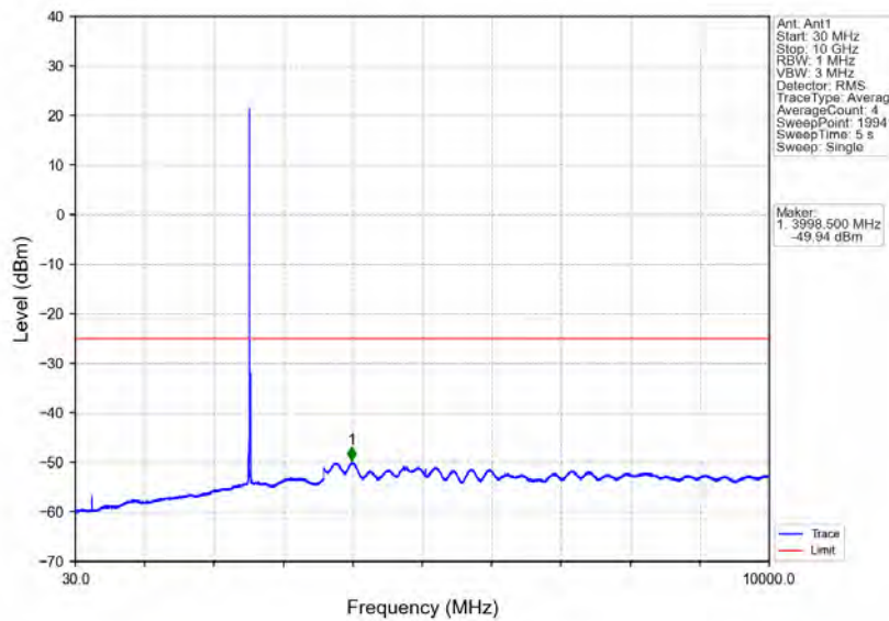
Band7_10MHz_QPSK_MCH_2535MHz_RB_1_0_NTNV
