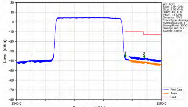
Band7_20MHz_64QAM_HCH_2560MHz_RB_100_0_NTNV
