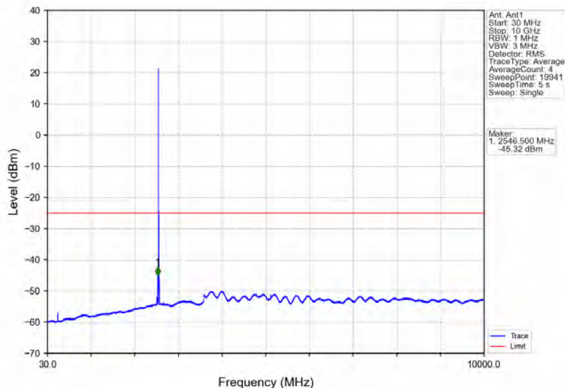
Band7_5MHz_QPSK_HCH_2567.5MHz_RB_1_0_NTNV
