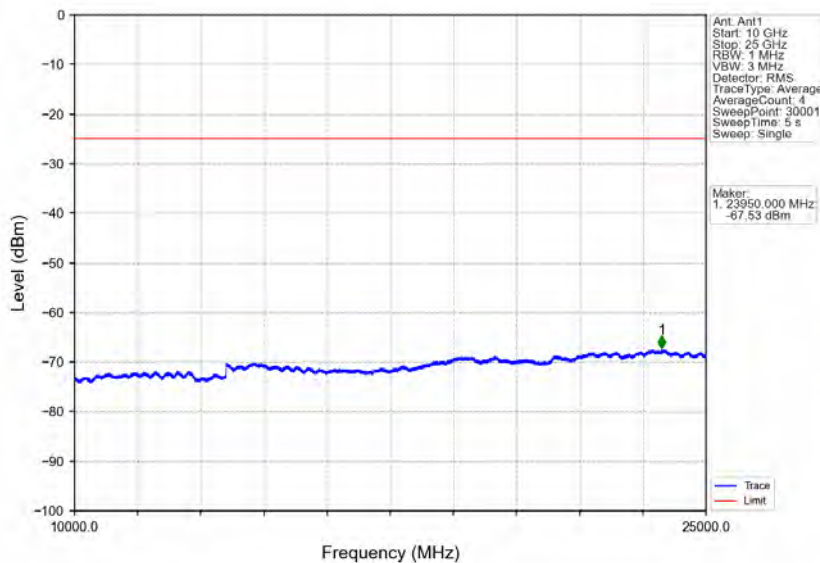
Band7_10MHz_QPSK_HCH_2565MHz_RB_1_0_NTNV
