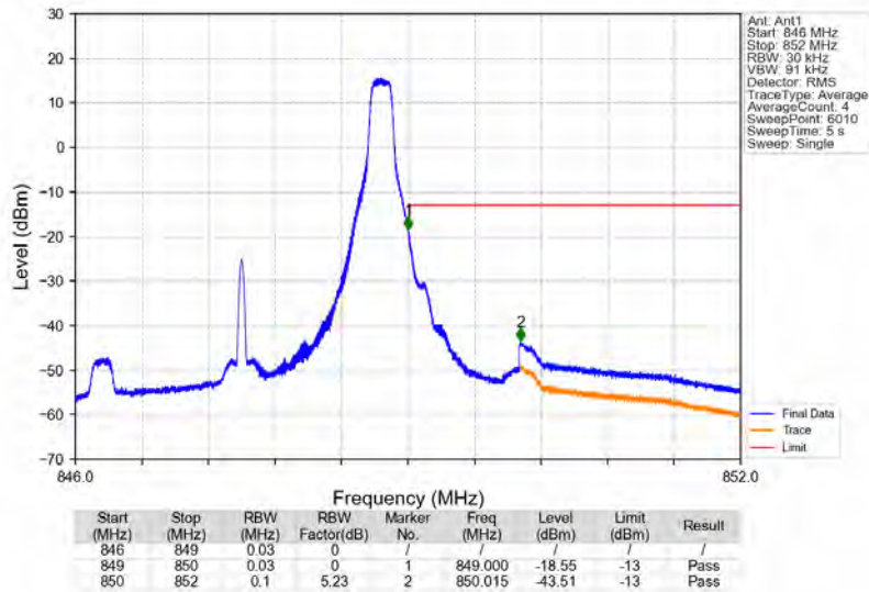
Band5_3MHz_QPSK_HCH_847.5MHz_RB_1_14_NTNV
