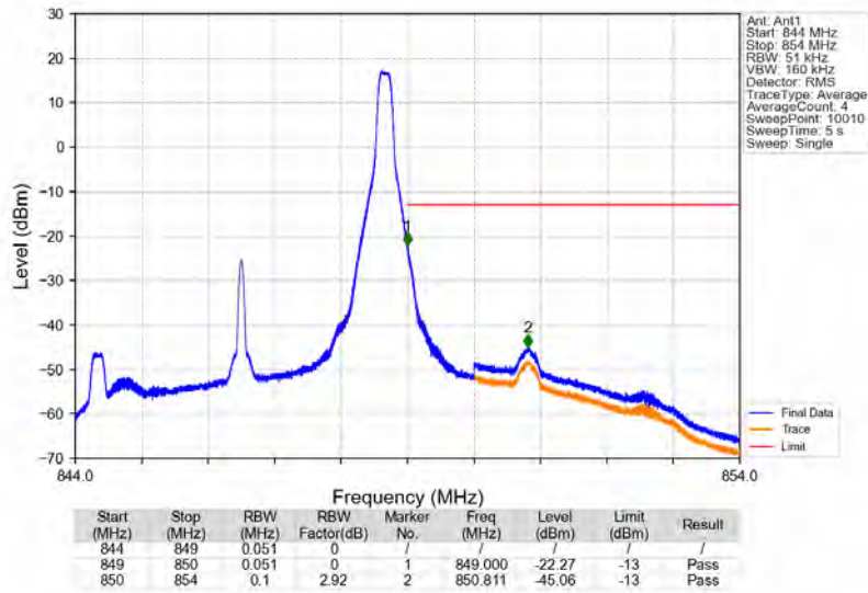
Band5_5MHz_QPSK_HCH_846.5MHz_RB_1_24_NTNV
