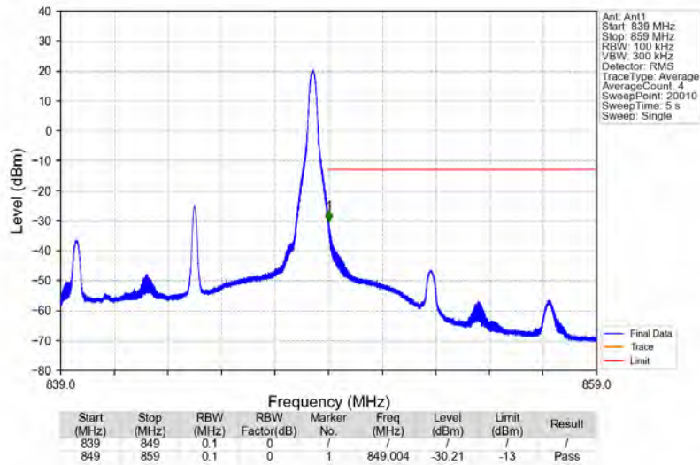
Band5_10MHz_QPSK_HCH_844MHz_RB_1_49_NTNV
