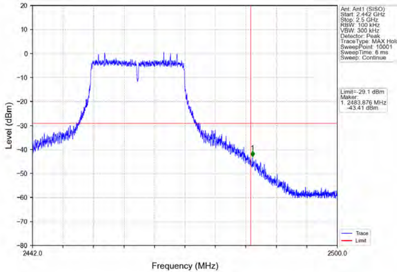
802.11n(HT20) HCH 2462MHz Ant1 (SISO) NTV
