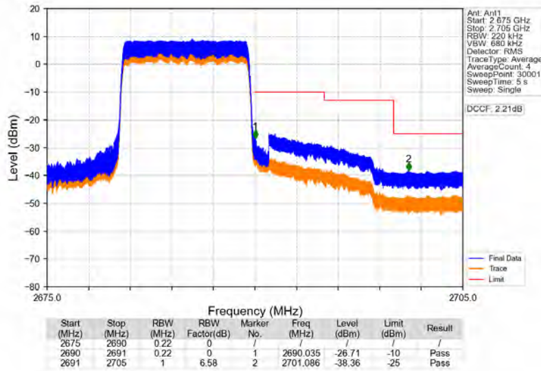
Band41_10MHz_QPSK_HCH_2685MHz_RB_50_0_NTV
