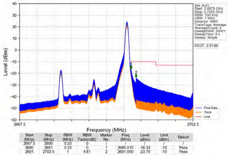
Band41_15MHz_QPSK_HCH_2682.5MHz_RB_1_74_NTNV
