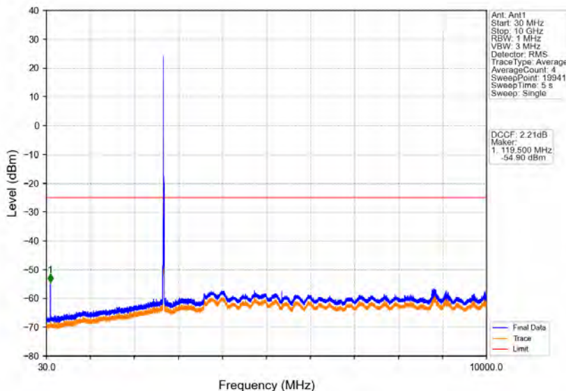
Band41_10MHz_QPSK_HCH_2685MHz_RB_1_0_NTNV
