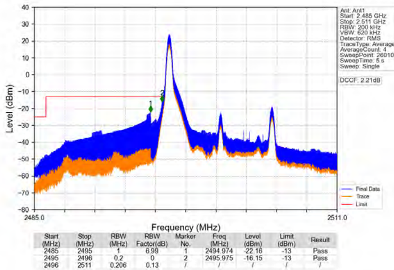
Band41_10MHz_16QAM_LCH_2501MHz_RB_1_0_NTV
