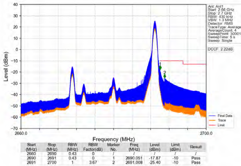
Band41_20MHz_QPSK_HCH_2680MHz_RB_1_99_NTNV
