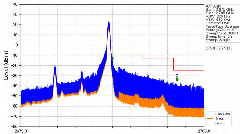
Band41_10MHz_64QAM_HCH_2685MHz_RB_1_49_NTNV
