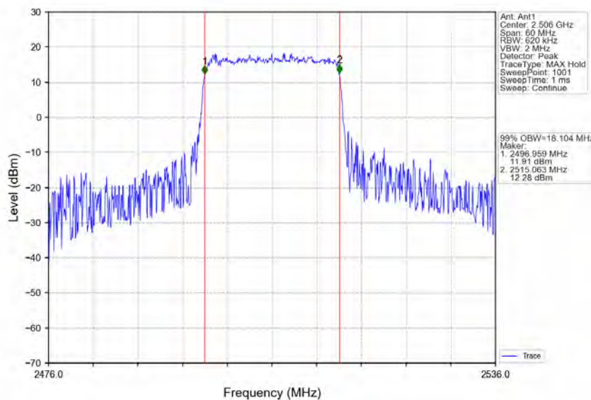
Band41_20MHz_QPSK_LCH_2506MHz_RB_100_0_NTNV
