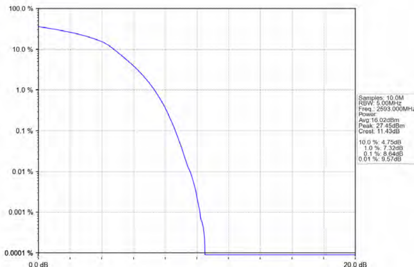
Band41_10MHz_64QAM_MCH_2593MHz_RB_50_0_NTNV
