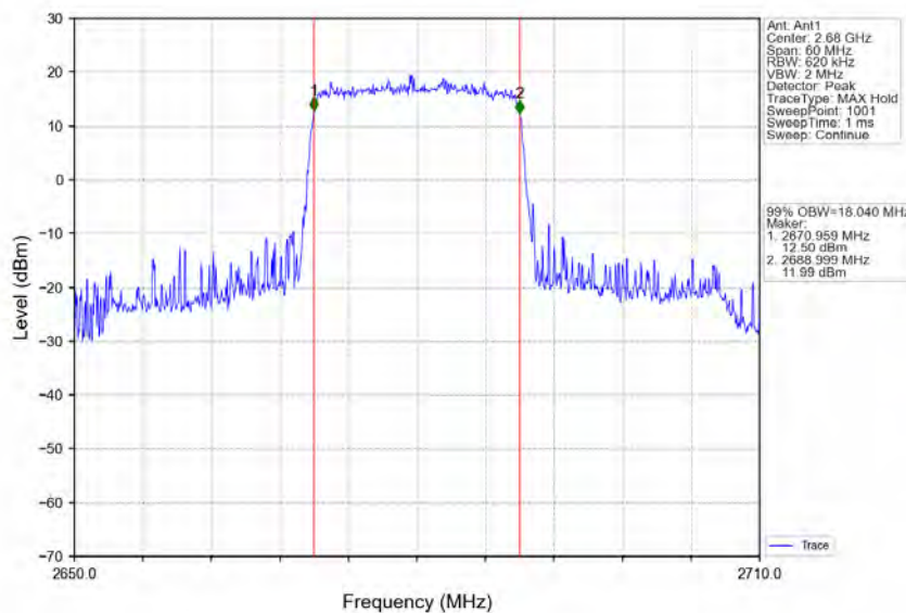
Band41_20MHz_QPSK_HCH_2680MHz_RB_100_0_NTNV
