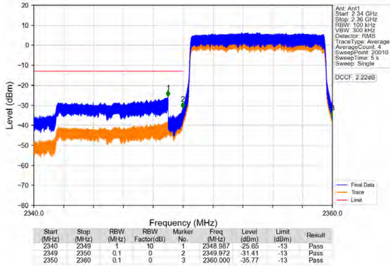
Band40b_10MHz_QPSK_LCH_2355MHz_RB_50_0_NTNV
