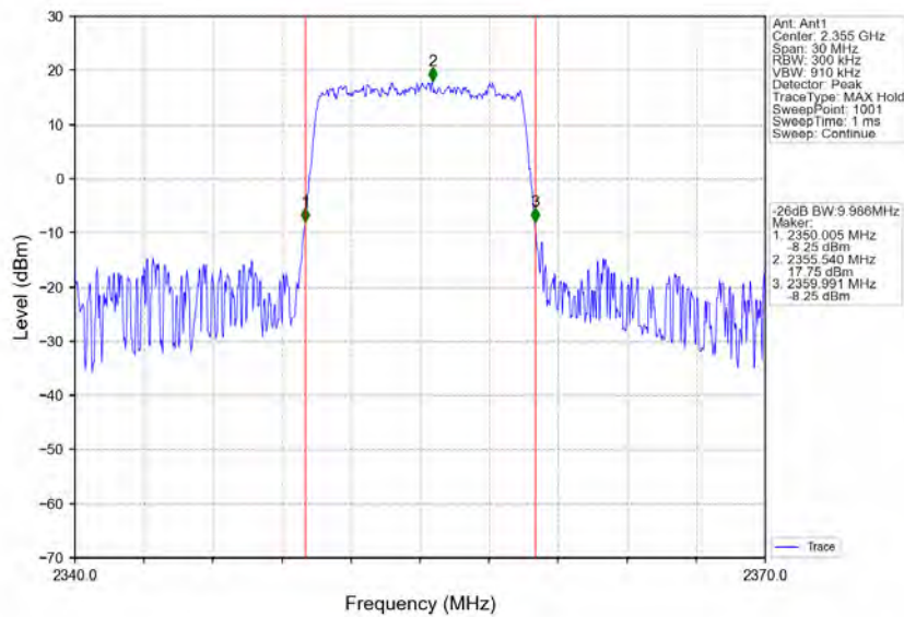
Band40b_10MHz_16QAM_MCH_2355MHz_RB_50_0_NTNV
