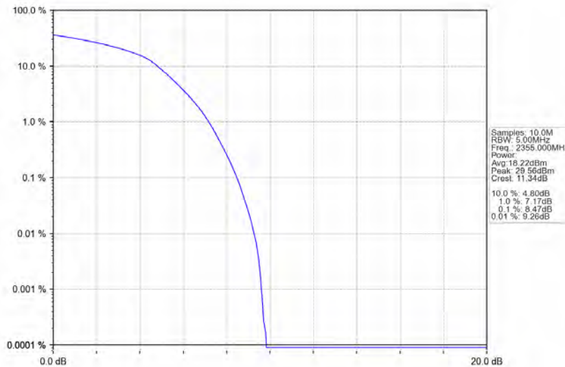
Band40b_10MHz_16QAM_LCH_2355MHz_RB_50_0_NTNV
