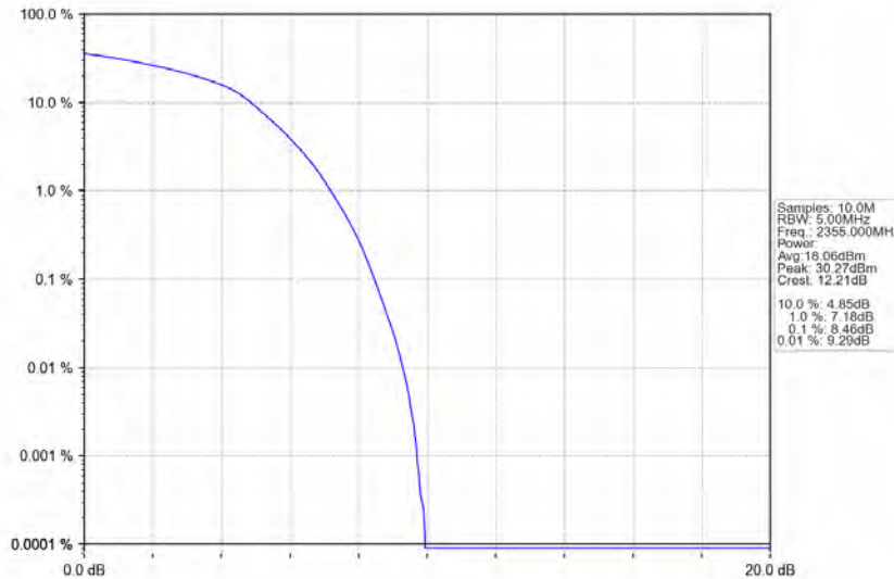
Band40b_10MHz_16QAM_MCH_2355MHz_RB_50_0_NTNV
