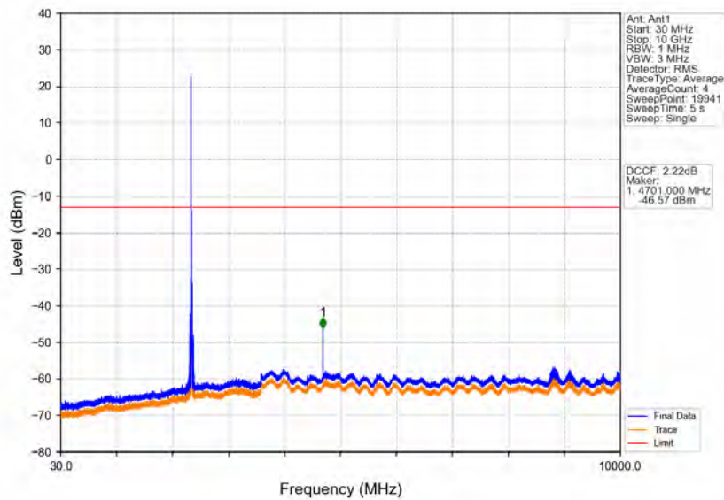
Band40b_10MHz_QPSK_HCH_2355MHz_RB_1_0_NTV
