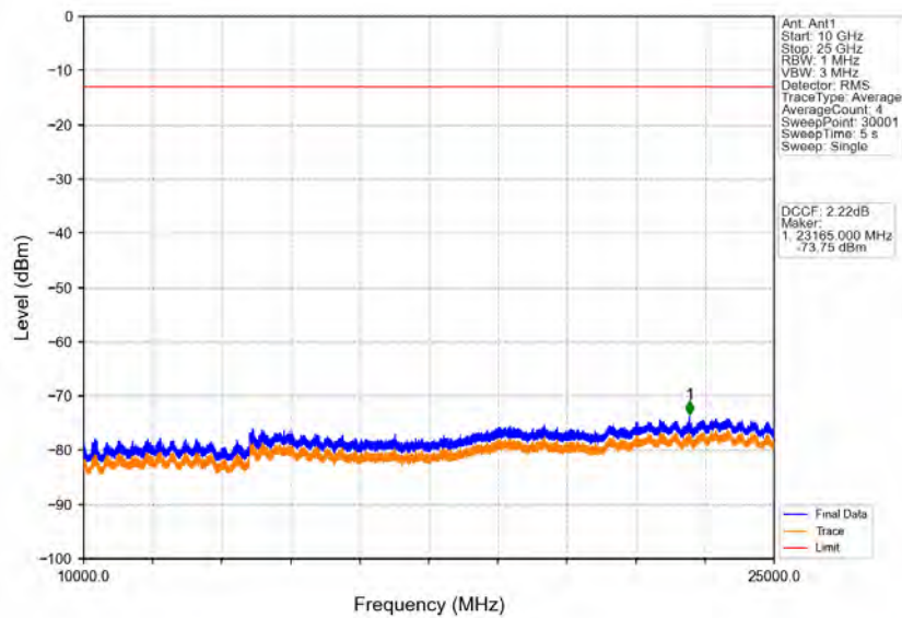
Band40b_10MHz_QPSK_HCH_2355MHz_RB_1_0_NTV
