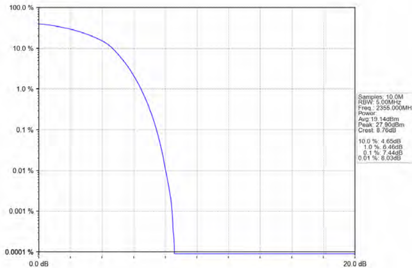
Band40b_10MHz_QPSK_HCH_2355MHz_RB_50_0_NTNV
