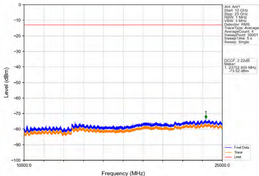
Band40b_10MHz_QPSK_LCH_2355MHz_RB_1_0_NTNV
