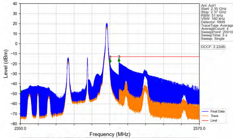
Band40b_5MHz_QPSK_HCH_2357.5MHz_RB_1_24_NTNV
