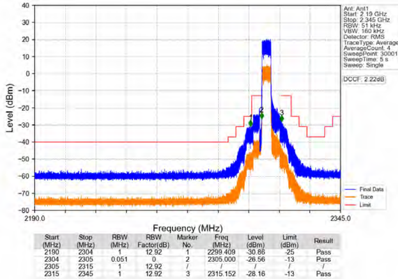
Band40a_5MHz_QPSK_MCH_2310MHz_RB_1_0_NTNV
