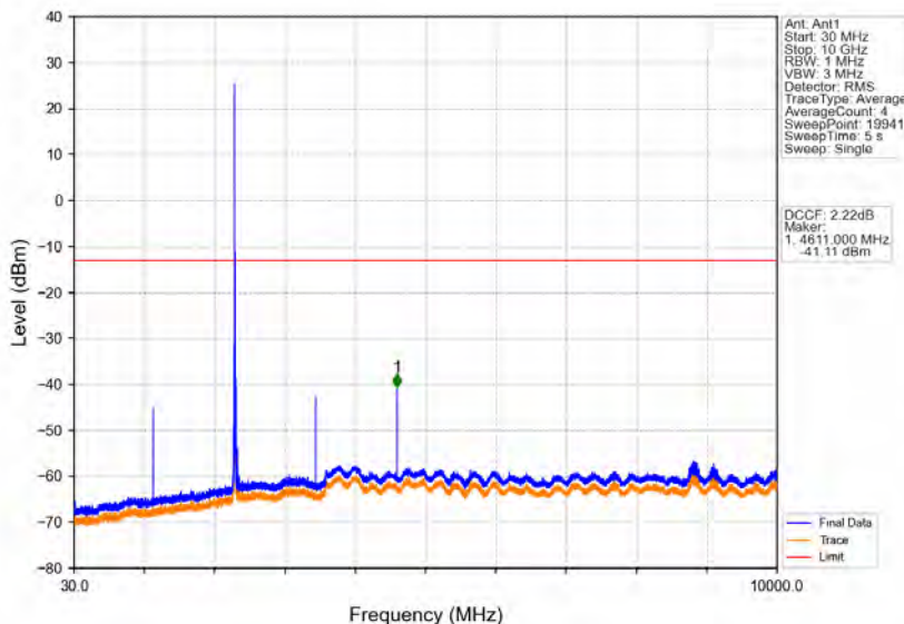
Band40a_10MHz_QPSK_HCH_2310MHz_RB_1_0_NTV
