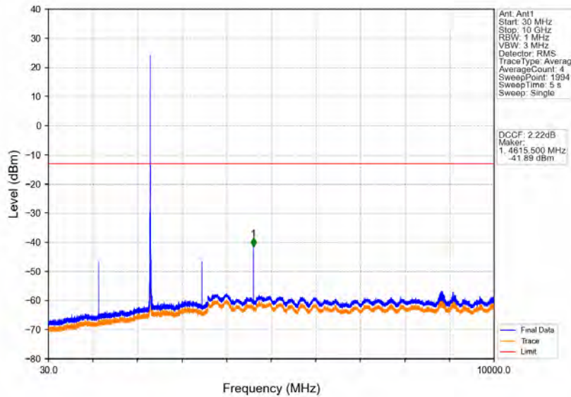
Band40a_5MHz_QPSK_MCH_2310MHz_RB_1_0_NTNV
