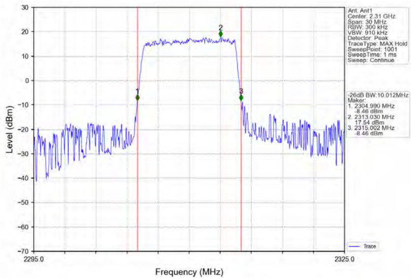
Band40a_10MHz_16QAM_MCH_2310MHz_RB_50_0_NTNV
