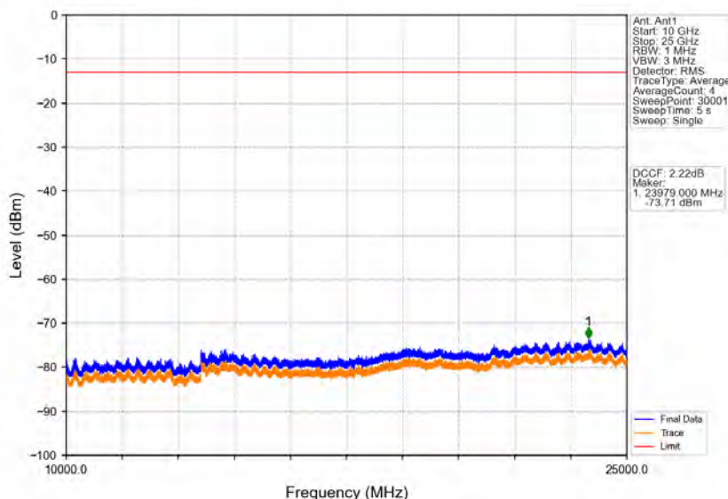
Band40a_10MHz_QPSK_HCH_2310MHz_RB_1_0_NTV
