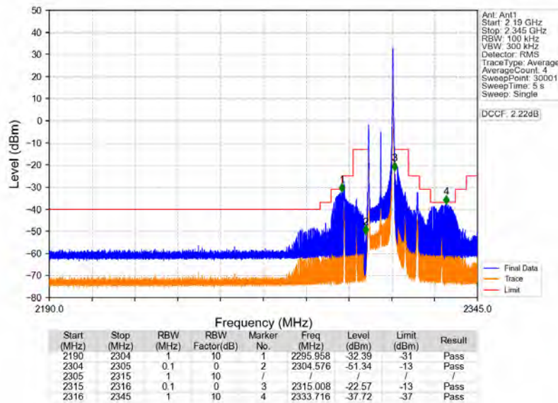
Band40a_10MHz_QPSK_HCH_2310MHz_RB_1_49_NTNV
