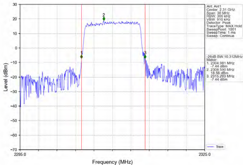
Band40a_10MHz_QPSK_LCH_2310MHz_RB_50_0_NTNV
