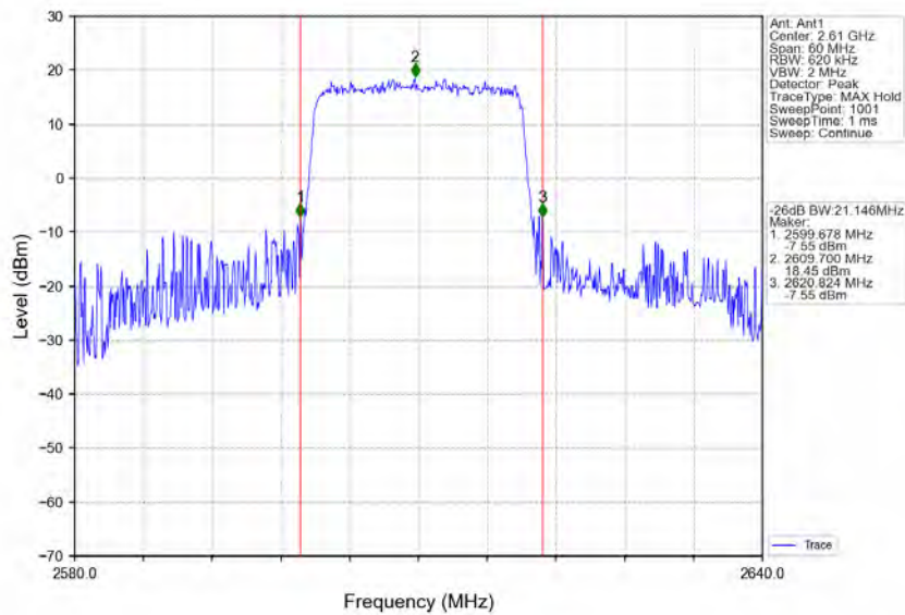
Band38_20MHz_QPSK_HCH_2610MHz_RB_100_0_NTNV
