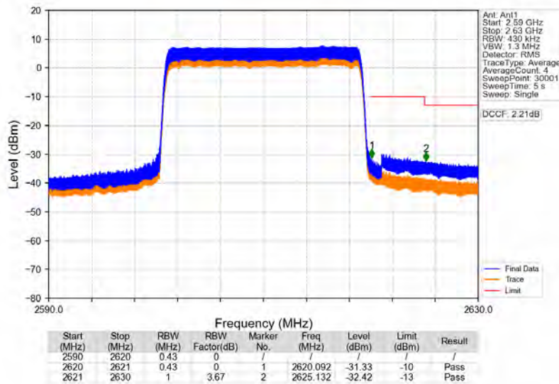
Band38_20MHz_16QAM_HCH_2610MHz_RB_100_0_NTNV
