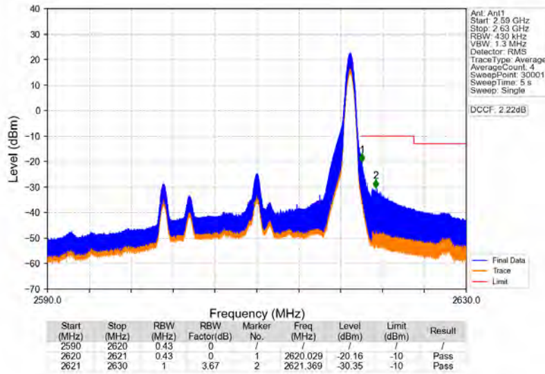
Band38_20MHz_64QAM_HCH_2610MHz_RB_1_99_NTNV
