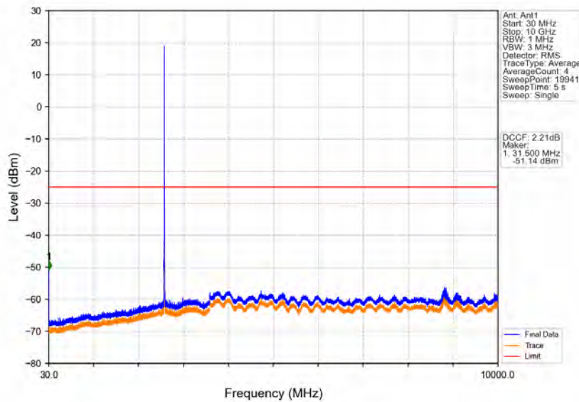
Band38_5MHz_QPSK_MCH_2595MHz_RB_1_0_NTNV
