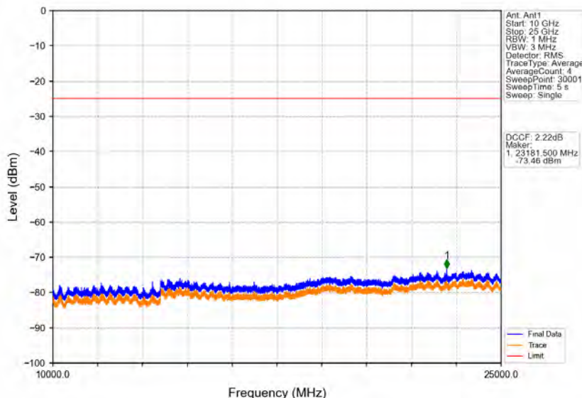
Band38_20MHz_16QAM_MCH_2595MHz_RB_1_0_NTNV
