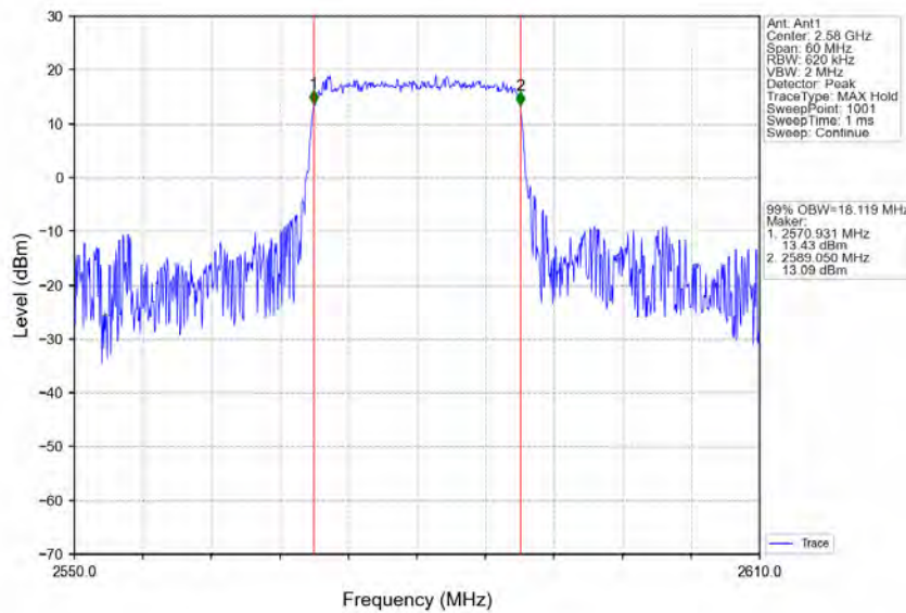
Band38_20MHz_QPSK_LCH_2580MHz_RB_100_0_NTNV
