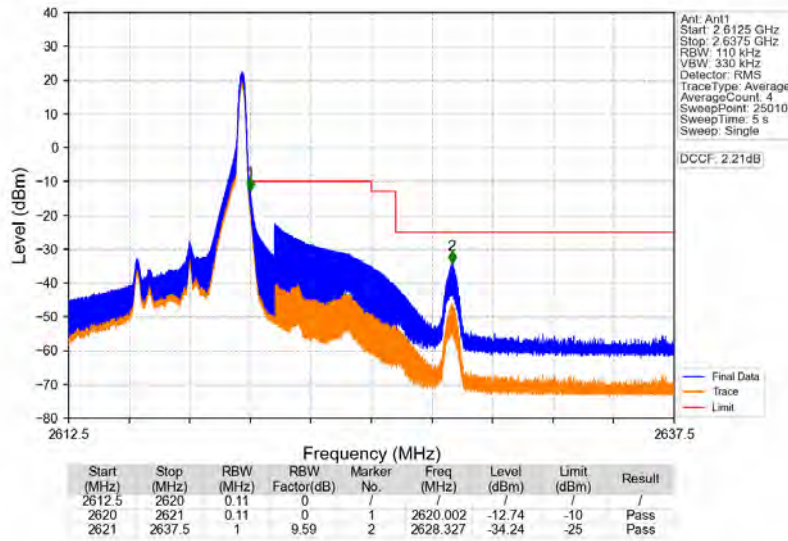
Band38_5MHz_QPSK_HCH_2617.5MHz_RB_1_24_NTNV
