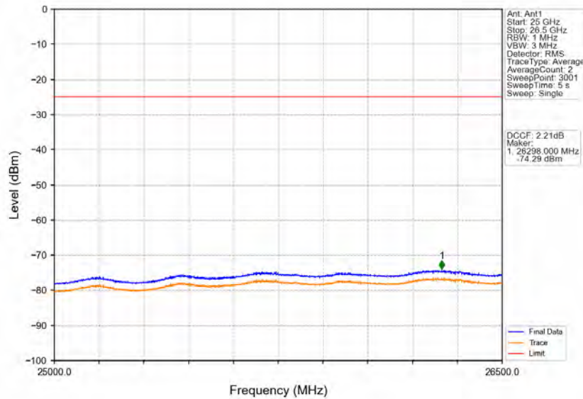
Band38_5MHz_QPSK_HCH_2617.5MHz_RB_1_24_NTNV
