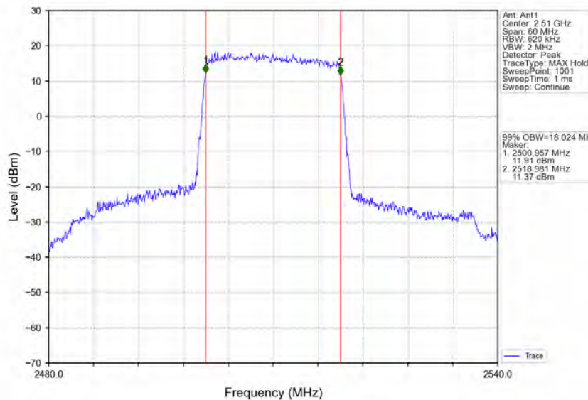
Band7_20MHz_QPSK_LCH_2510MHz_RB_100_0_NTNV
