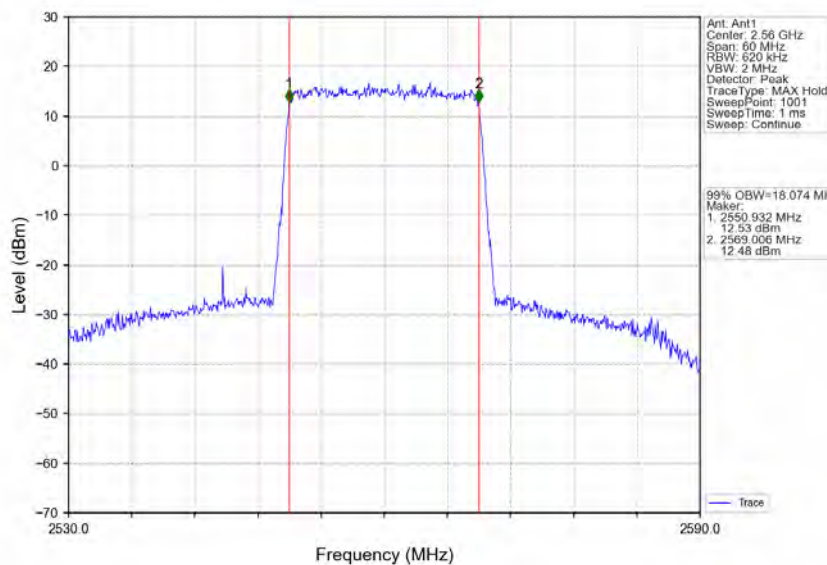
Band7_20MHz_64QAM_HCH_2560MHz_RB_100_0_NTNV
