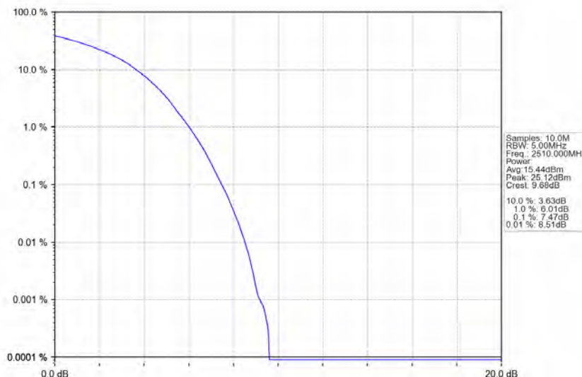
Band7_20MHz_64QAM_LCH_2510MHz_RB_100_0_NTNV
