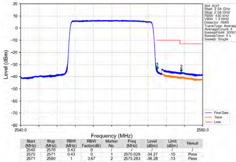
Band7_20MHz_QPSK_HCH_2560MHz_RB_100_0_NTNV
