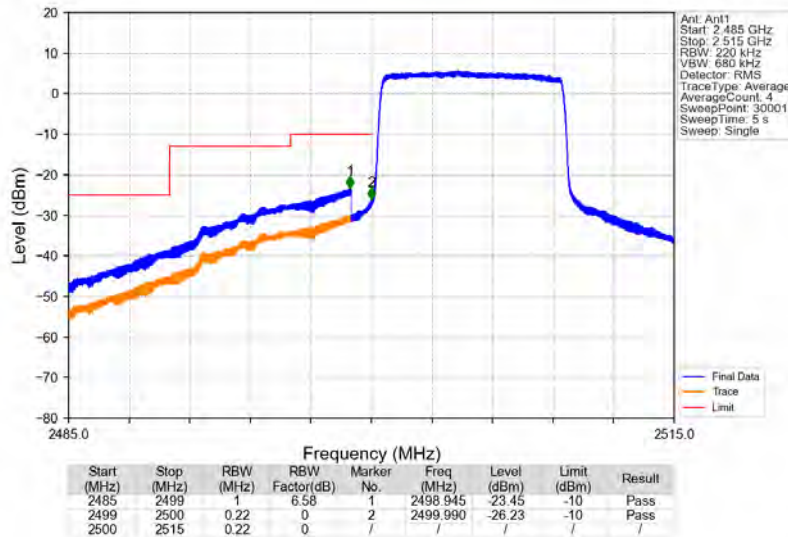
Band7_10MHz_QPSK_LCH_2505MHz_RB_50_0_NTNV
