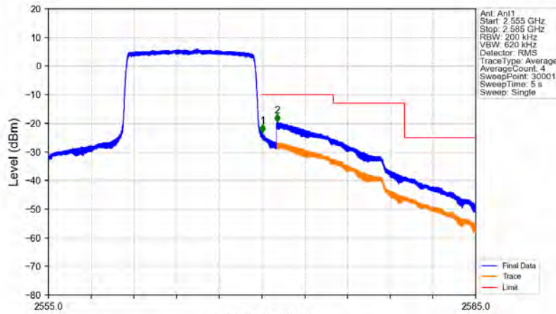
Band7_10MHz_QPSK_HCH_2565MHz_RB_50_0_NTNV
