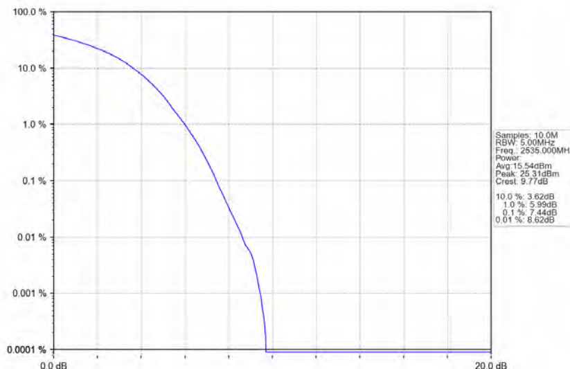
Band7_20MHz_64QAM_MCH_2535MHz_RB_100_0_NTNV
