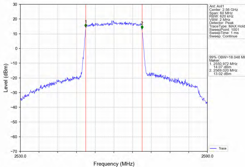
Band7_20MHz_QPSK_HCH_2560MHz_RB_100_0_NTNV
