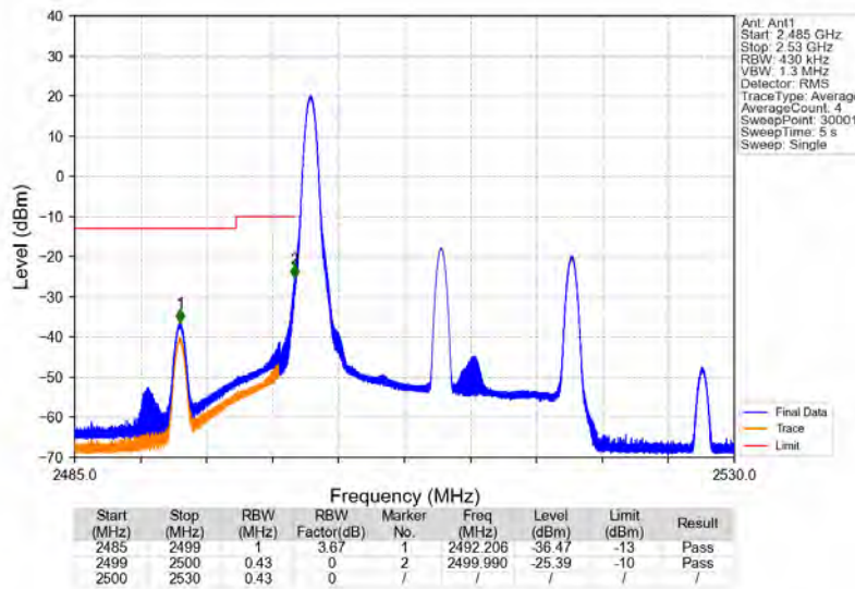
Band7_20MHz_16QAM_LCH_2510MHz_RB_1_0_NTNV
