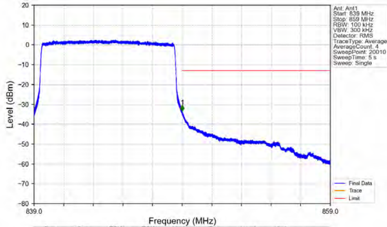
Band5_10MHz_QPSK_HCH_844MHz_RB_50_0_NTNV
