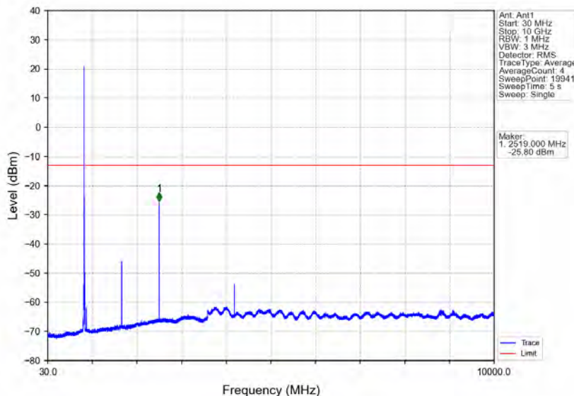
Band5_10MHz_QPSK_HCH_844MHz_RB_1_49_NTNV
