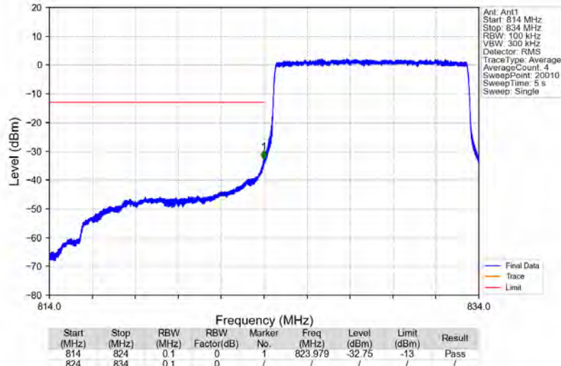
Band5_10MHz_QPSK_LCH_829MHz_RB_50_0_NTNV
