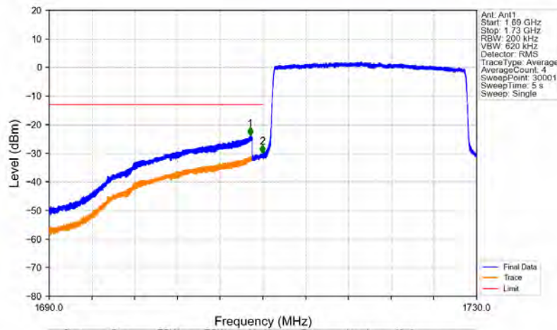
Band4_20MHz_16QAM_LCH_1720MHz_RB_100_0_NTNV
