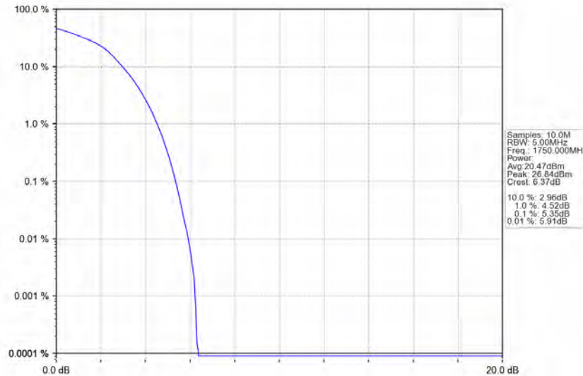
Band4_10MHz_QPSK_HCH_1750MHz_RB_50_0_NTNV
