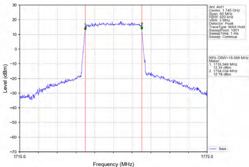
Band4_20MHz_QPSK_HCH_1745MHz_RB_100_0_NTNV
