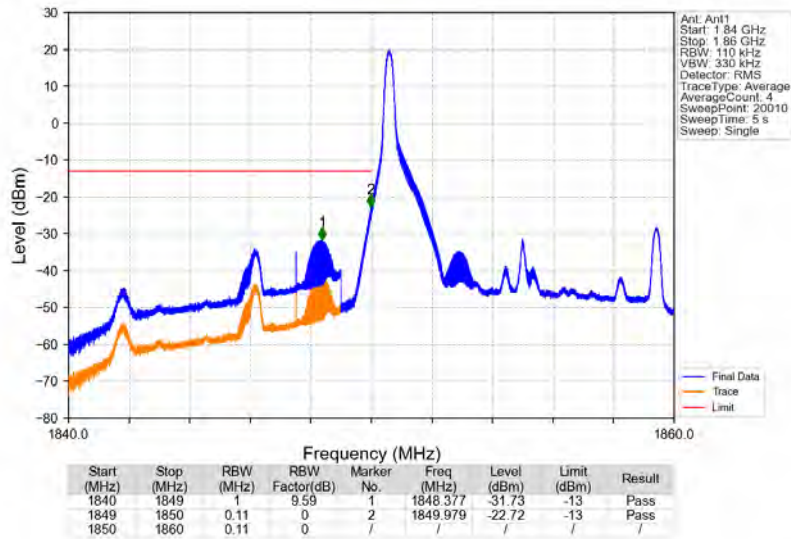
Band2_10MHz_64QAM_LCH_1855MHz_RB_1_0_NTNV
