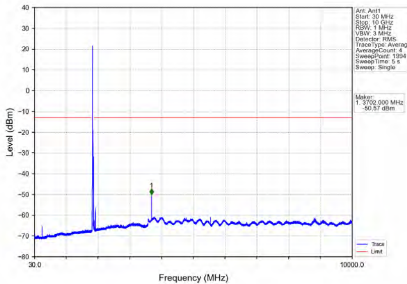
Band2_20MHz_16QAM_LCH_1860MHz_RB_1_0_NTNV
