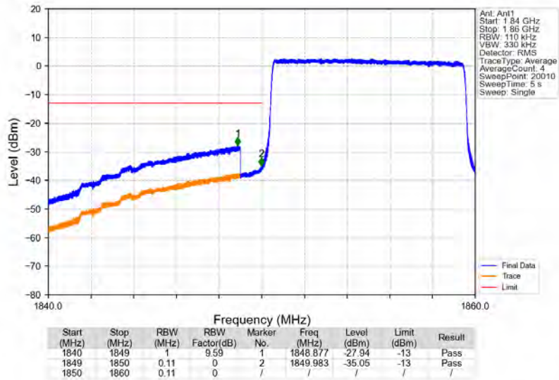
Band2_10MHz_64QAM_LCH_1855MHz_RB_50_0_NTV
