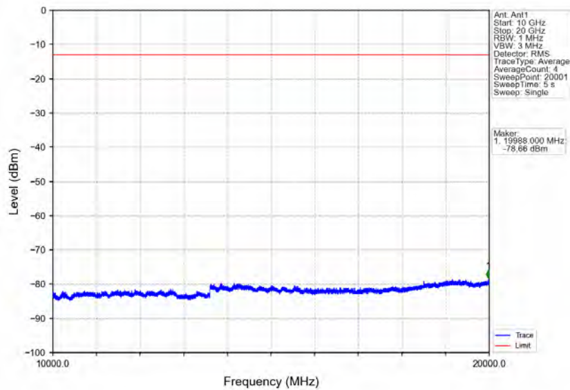
Band2_10MHz_64QAM_LCH_1855MHz_RB_50_0_NTV
