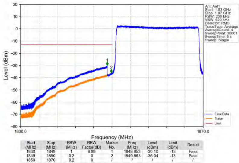
Band2_20MHz_64QAM_LCH_1860MHz_RB_100_0_NTNV
