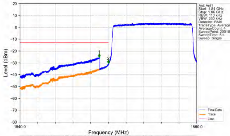
Band2_10MHz_QPSK_LCH_1855MHz_RB_50_0_NTNV
