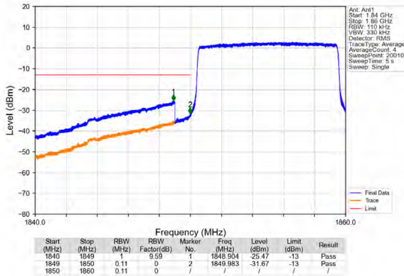
Band2_10MHz_16QAM_LCH_1855MHz_RB_50_0_NTV
