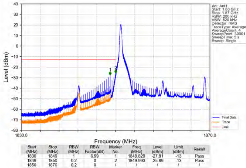
Band2_20MHz_64QAM_LCH_1860MHz_RB_1_0_NTNV
