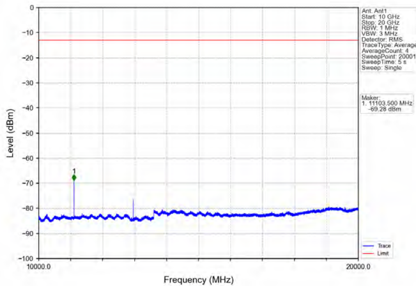
Band2_10MHz_16QAM_LCH_1855MHz_RB_50_0_NTV
