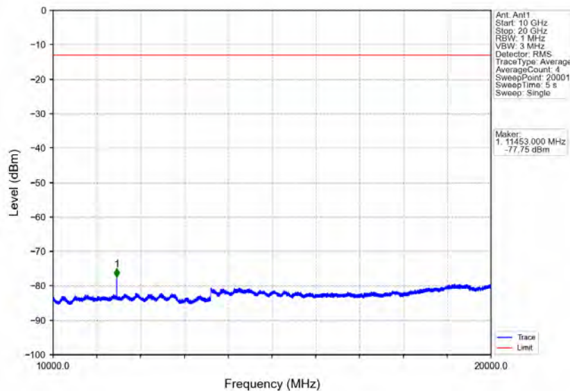
Band2_1.4MHz_QPSK_HCH_1909.3MHz_RB_1_0_NTV
