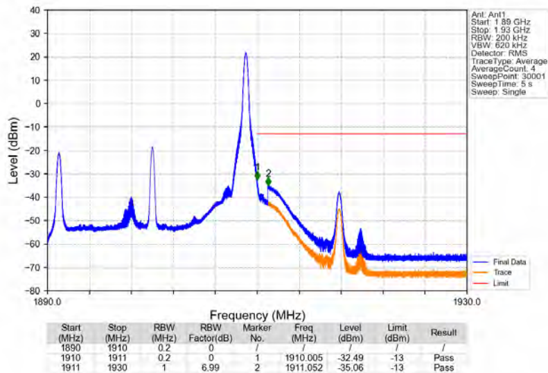
Band2_20MHz_QPSK_HCH_1900MHz_RB_1_99_NTNV
