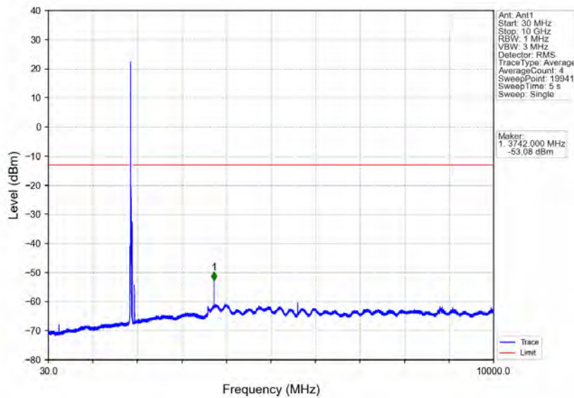
Band2_20MHz_QPSK_MCH_1880MHz_RB_1_0_NTNV
