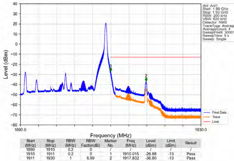
Band2_20MHz_64QAM_HCH_1900MHz_RB_1_99_NTNV
