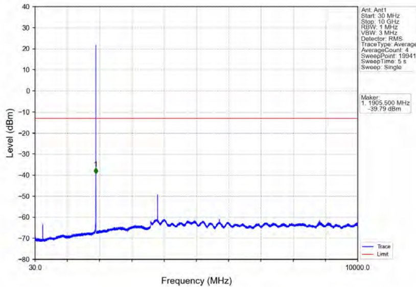
Band2_1.4MHz_QPSK_HCH_1909.3MHz_RB_1_0_NTV
