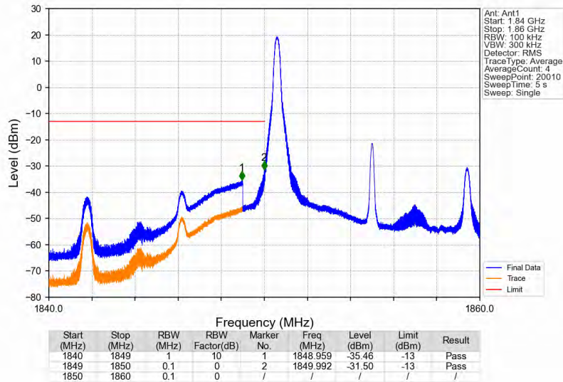
Band2_10MHz_16QAM_LCH_1855MHz_RB_1_0_NTNV
