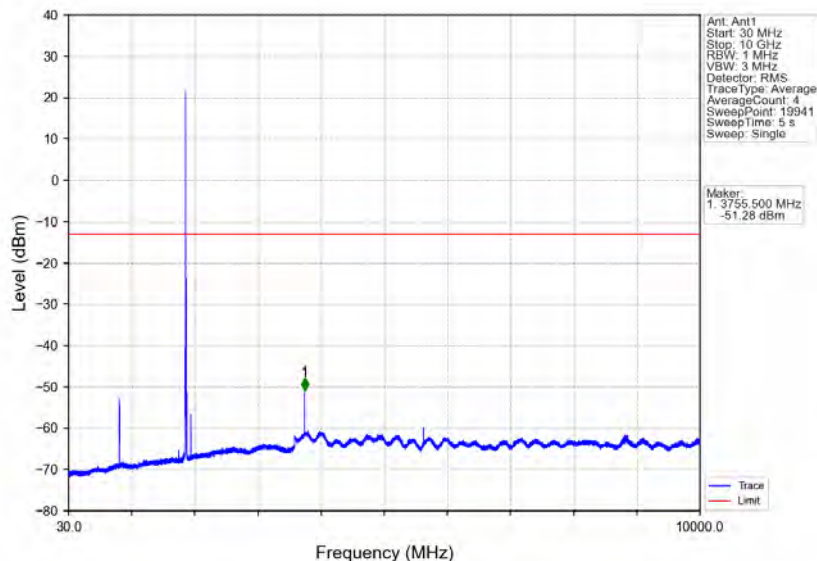
Band2_5MHz_QPSK_MCH_1880MHz_RB_1_0_NTNV
