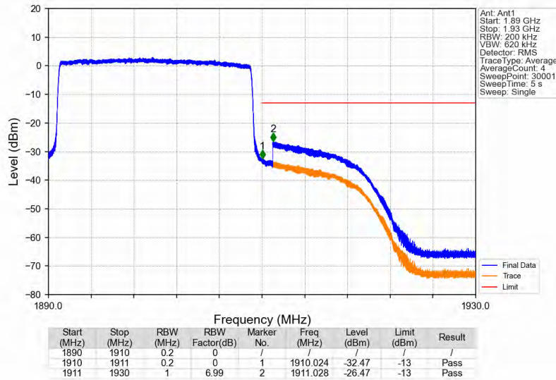
Band2_20MHz_16QAM_HCH_1900MHz_RB_100_0_NTNV
