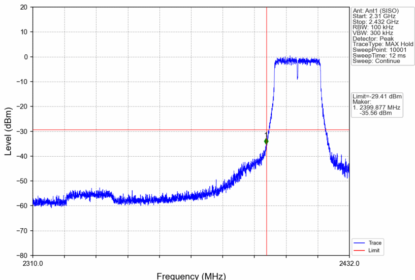
802.11n(HT20)_LCH_2412MHz_Ant1 (SISO)_NTNV
