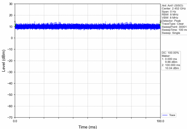
802.11n(HT40) HCH_2452MHz_Ant1 (SISO) NTVN
