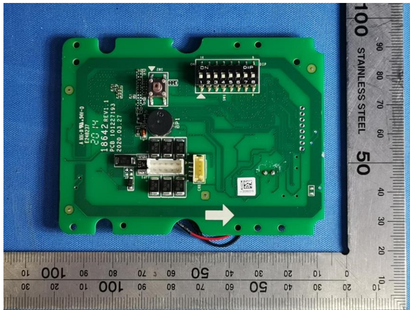
13.56MHz Module
