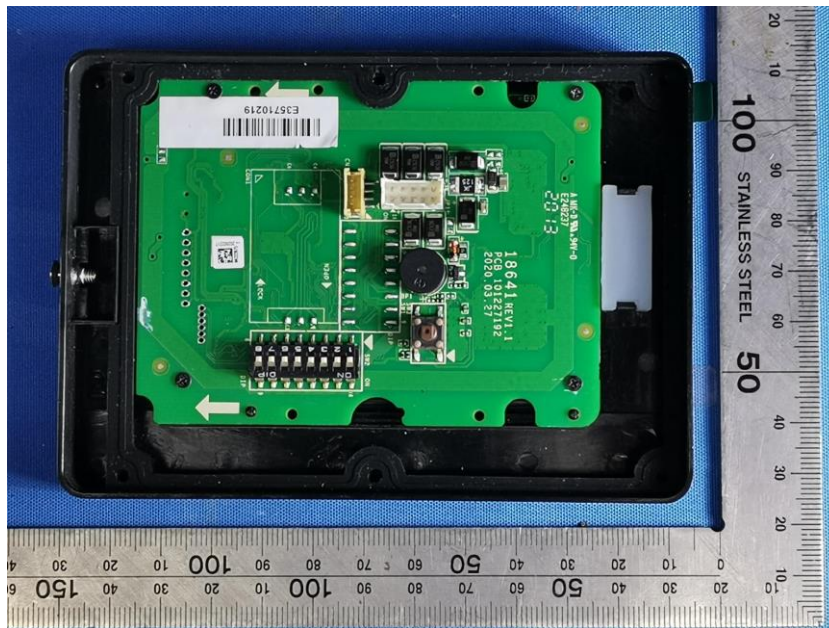
13.56MHz Module
