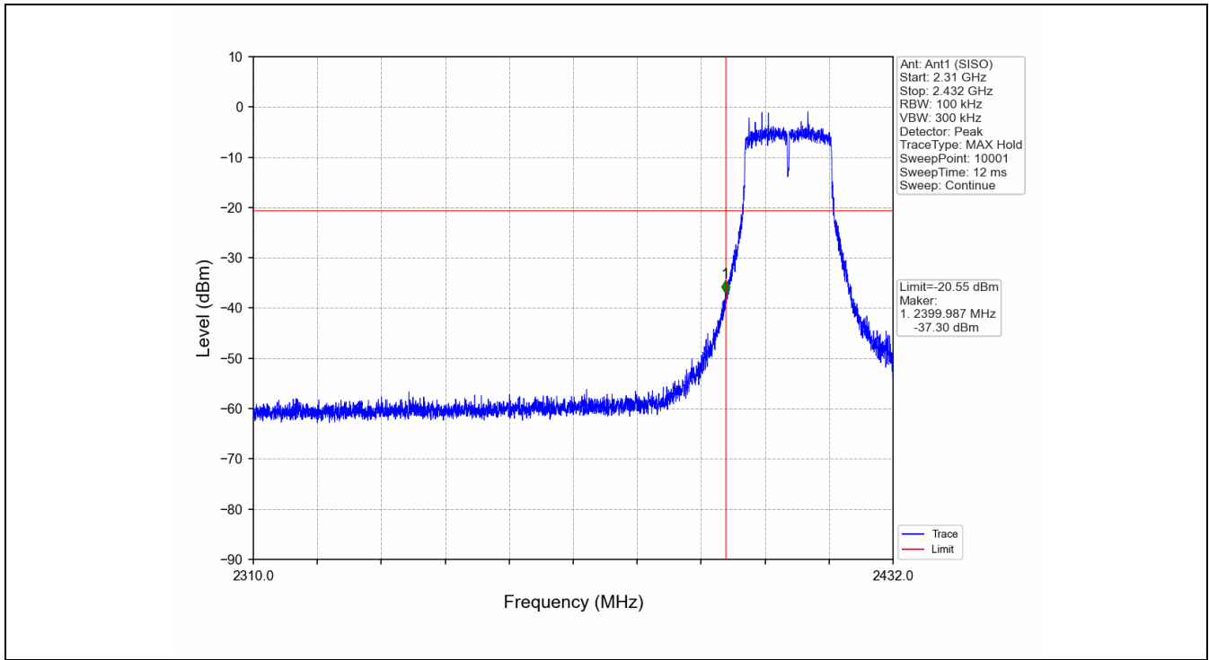
802.11g_LCH_2412MHz_Ant1 (SISO)_NTNV
