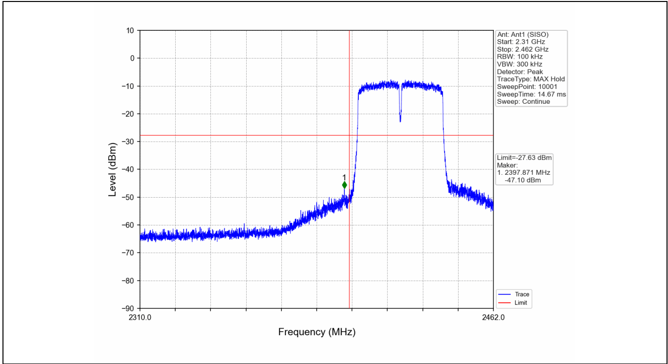
802.11n(HT40)_LCH_2422MHz_Ant1 (SISO)_NTNV
