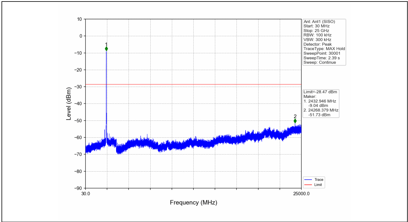
802.11n(HT40)_HCH_2452MHz_Ant1 (SISO)_NTNV
