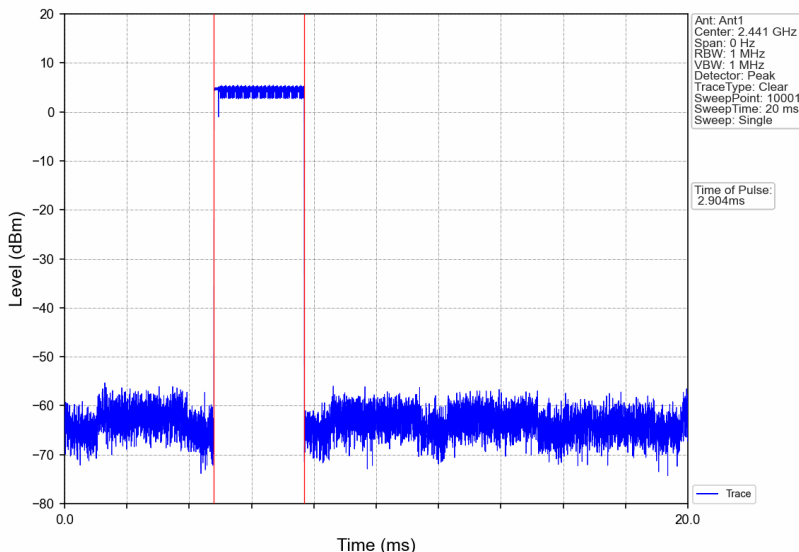
Pi/4DQPSK_2DH5_HOPP_Ant1_NTNV
