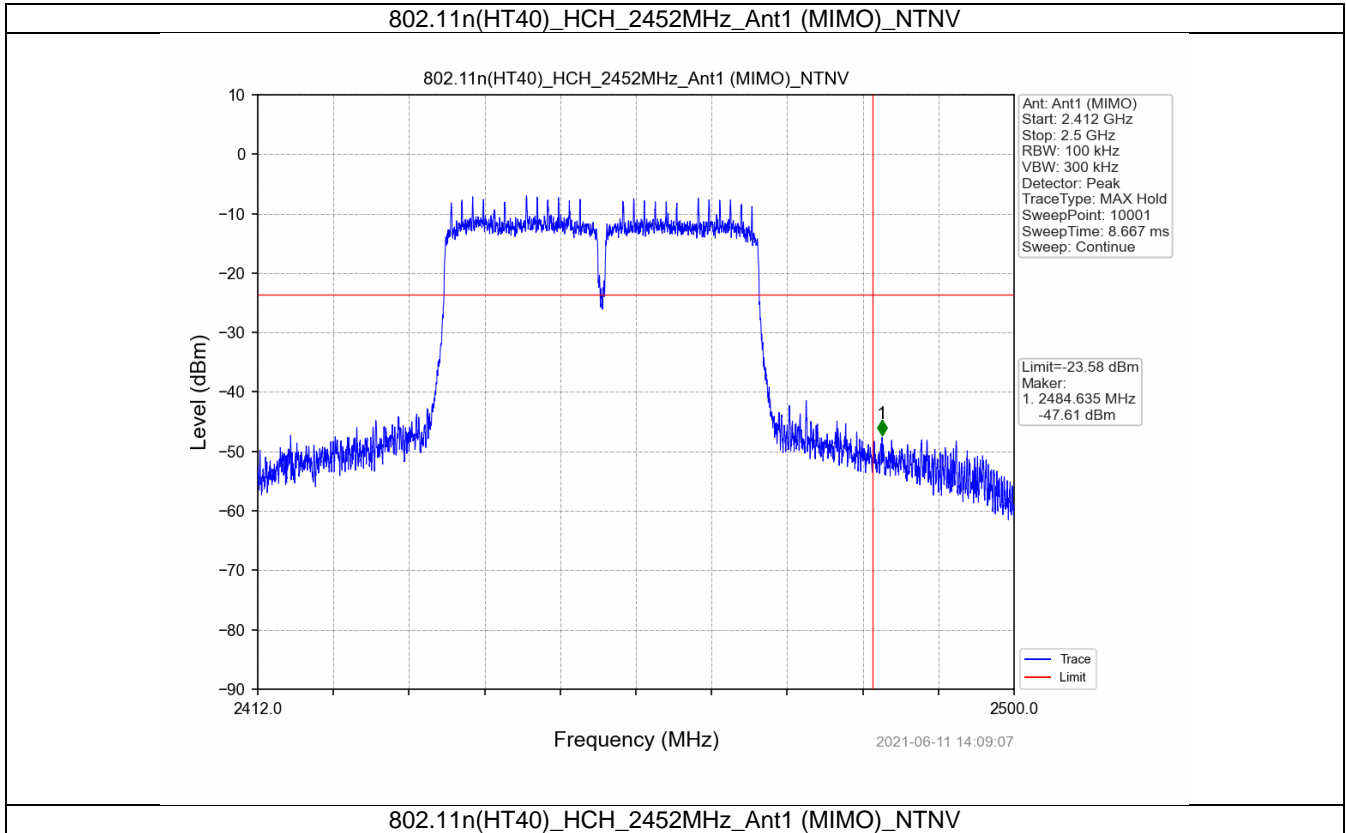
802.11n(HT40)_HCH_2452MHz_Ant1 (MIMO)_NTNV
