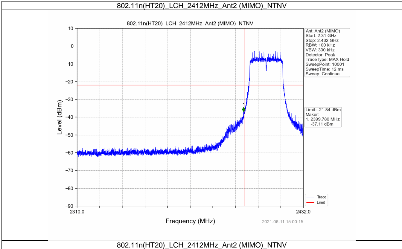
802.11n(HT20)_LCH_2412MHz_Ant2 (MIMO)_NTNV
