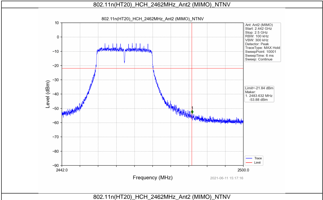
802.11n(HT20)_HCH_2462MHz_Ant2 (MIMO)_NTNV
