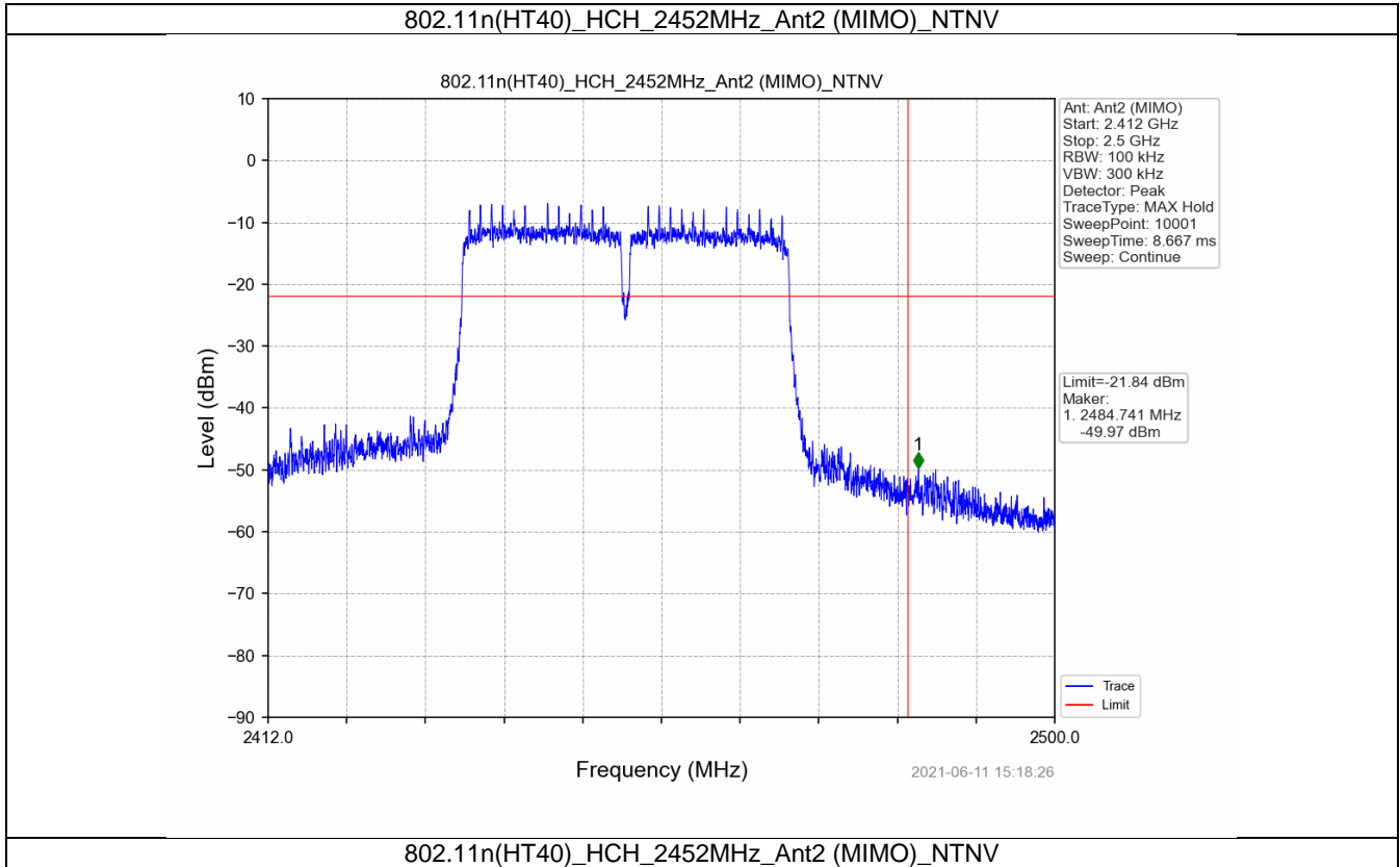
802.11n(HT40)_HCH_2452MHz_Ant2 (MIMO)_NTNV
