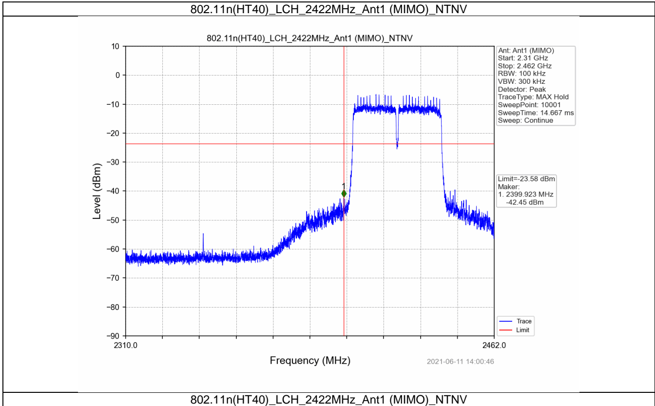
802.11n(HT40)_LCH_2422MHz_Ant1 (MIMO)_NTNV
