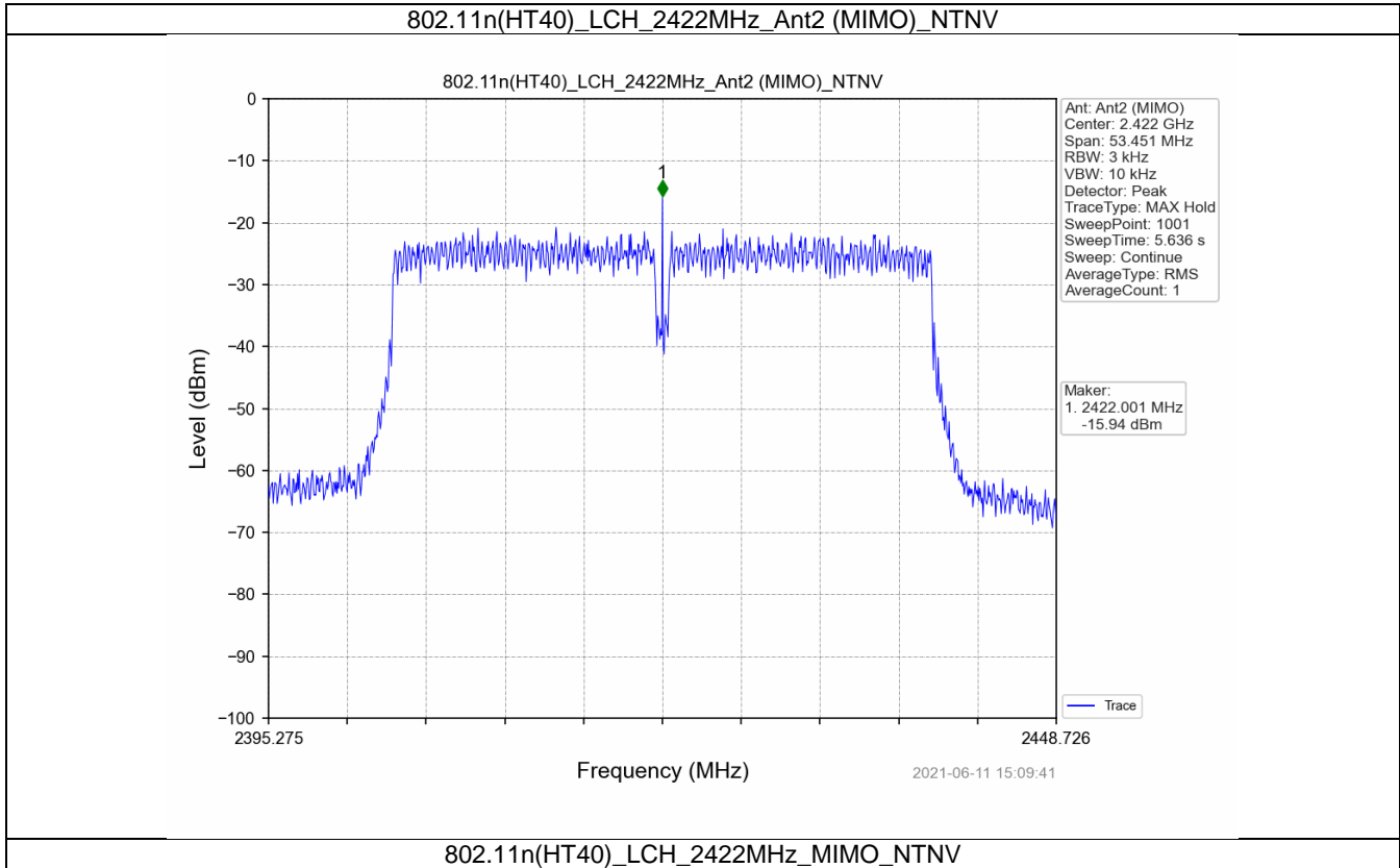
802.11n(HT40)_LCH_2422MHz_MIMO_NTNV
