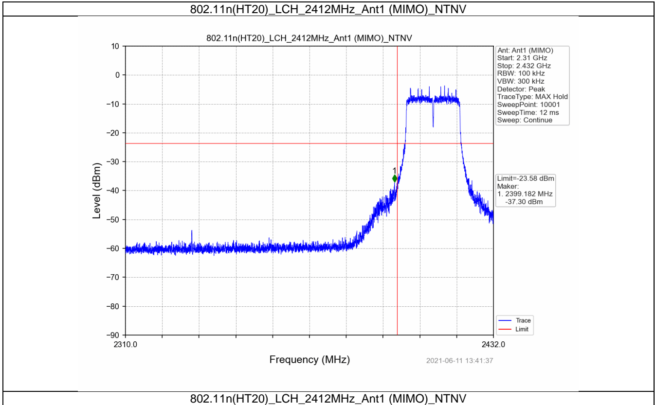
802.11n(HT20)_LCH_2412MHz_Ant1 (MIMO)_NTNV
