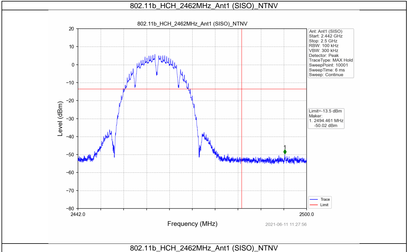
802.11b_HCH_2462MHz_Ant1 (SISO)_NTNV
