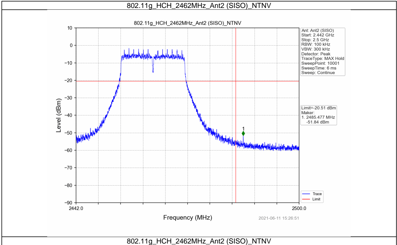
802.11g_HCH_2462MHz_Ant2 (SISO)_NTNV
