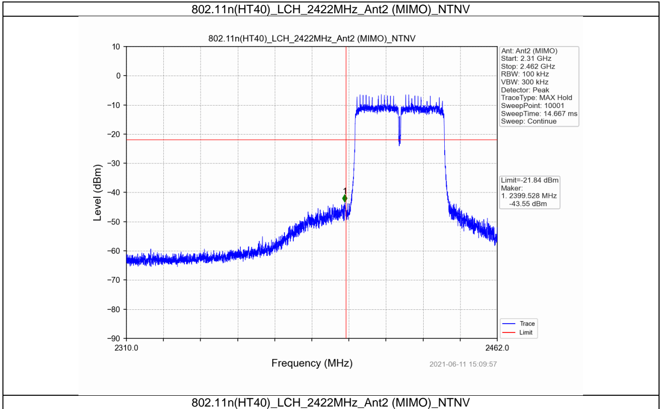
802.11n(HT40)_LCH_2422MHz_Ant2 (MIMO)_NTNV
