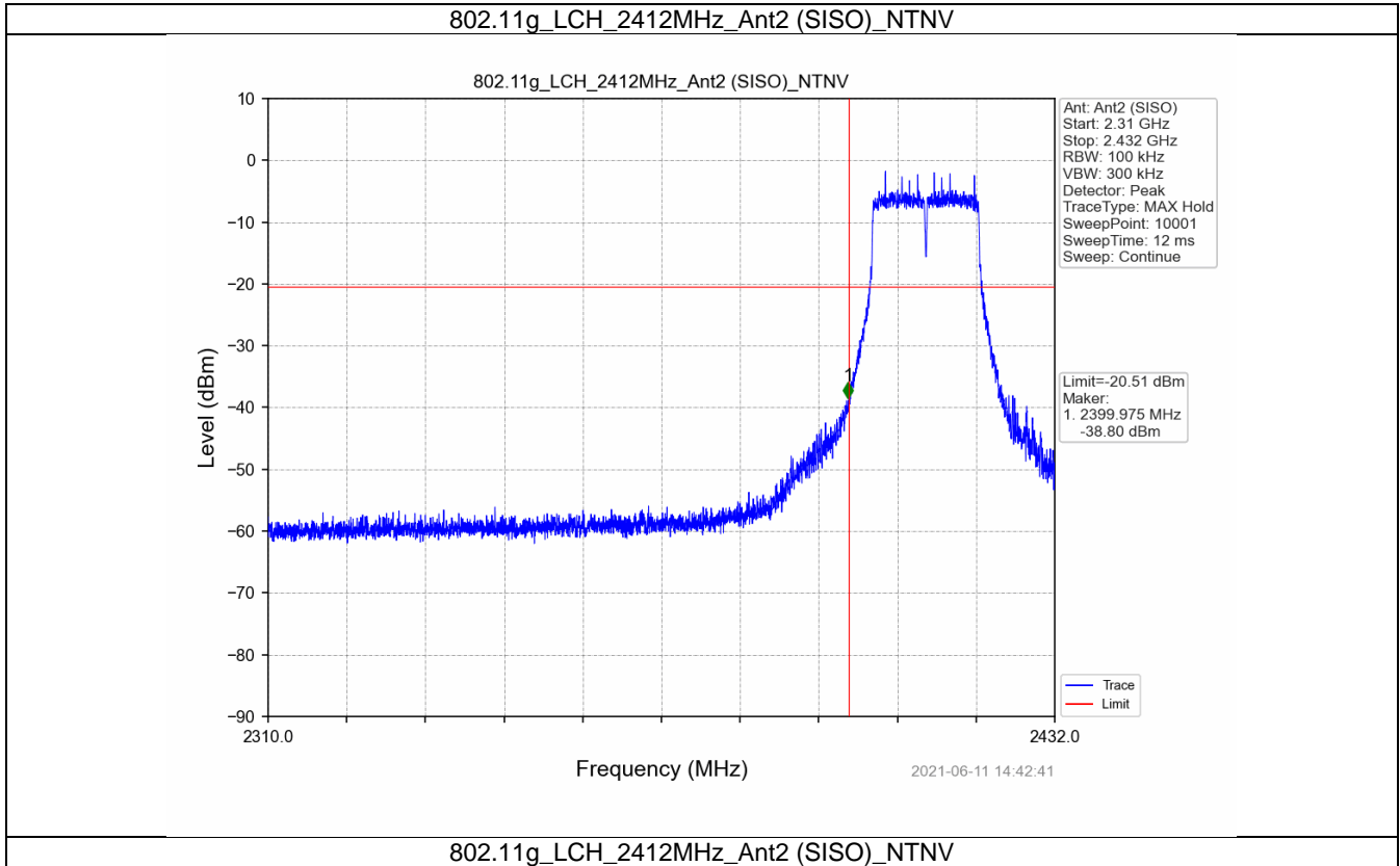
802.11g_LCH_2412MHz_Ant2 (SISO)_NTNV
