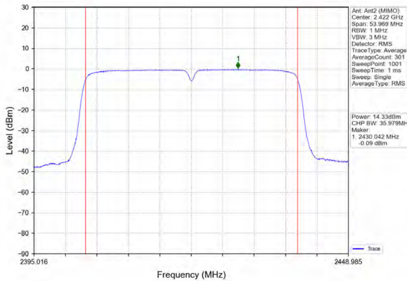
802.11n(HT40)_LCH_2422MHz_Ant2 (MIMO)_NTNV
