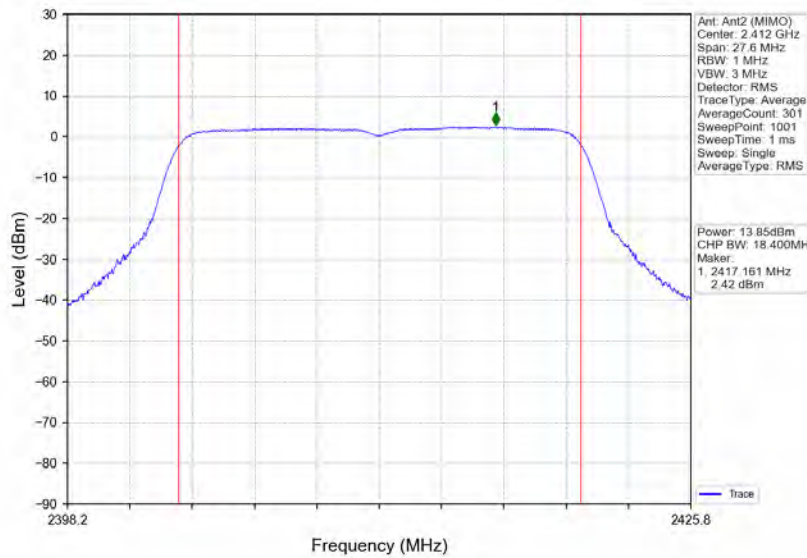
802.11n(HT20)_LCH_2412MHz_Ant2 (MIMO)_NTNV
