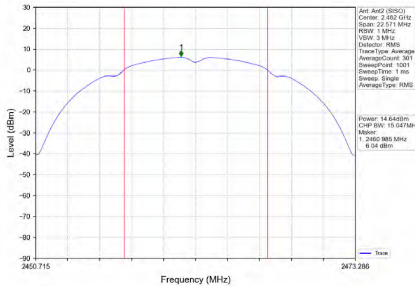
802.11b_HCH_2462MHz_Ant2 (SISO)_NTNV
