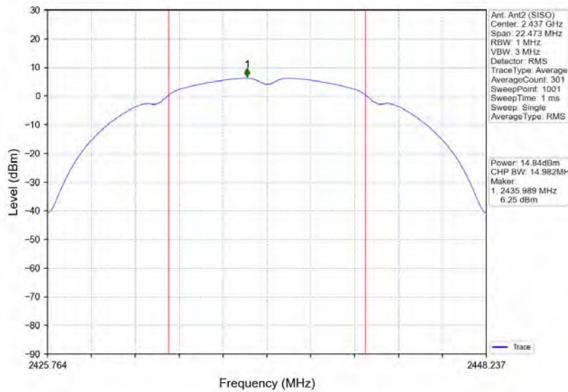
802.11b_MCH_2437MHz_Ant2 (SISO)_NTNV
