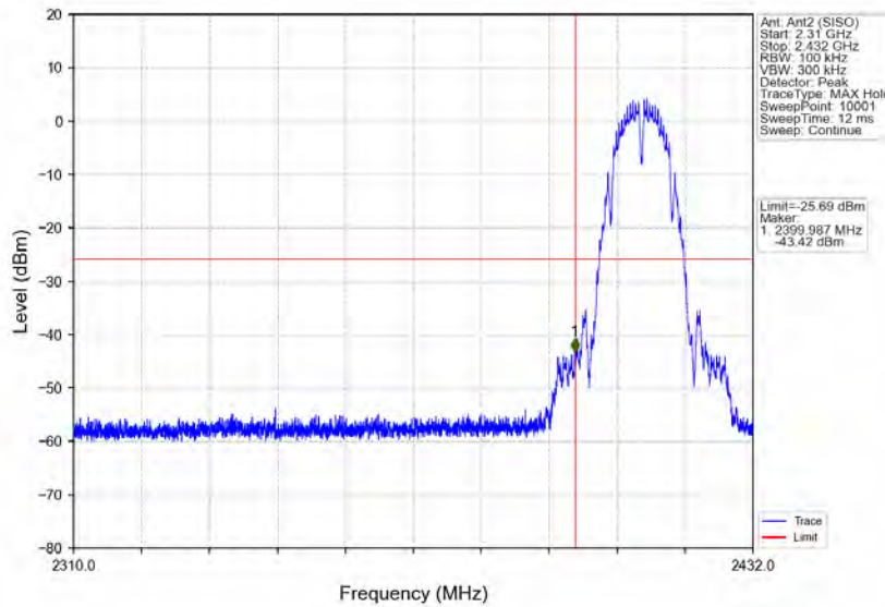
802.11b_LCH_2412MHz_Ant2 (SISO)_NTNV
