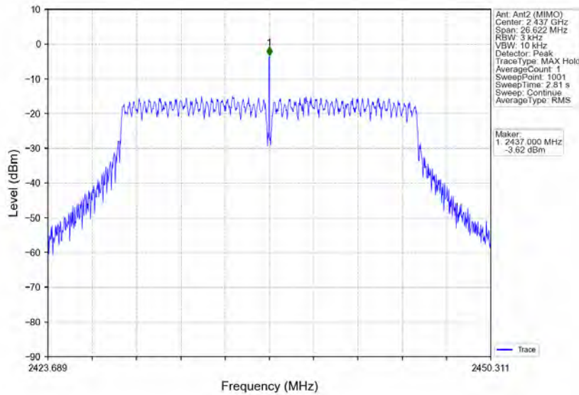
802.11n(HT20)_MCH_2437MHz_MIMO_NTNV
