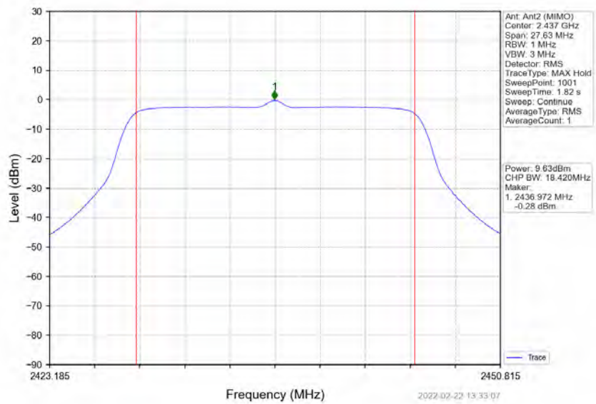
802.11n(HT20)_MCH_2437MHz_Ant2 (MIMO)_NTNV
