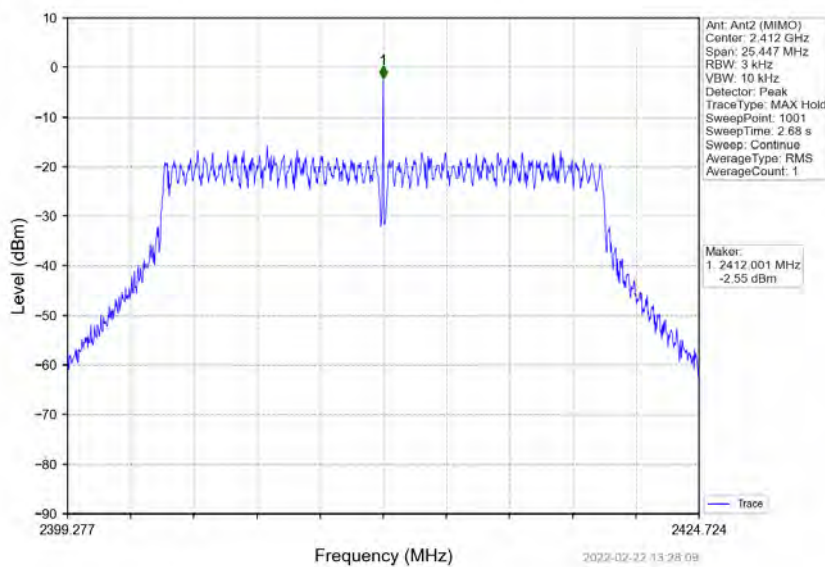
802.11n(HT20)_LCH_2412MHz_Ant2 (MIMO)_NTNV
