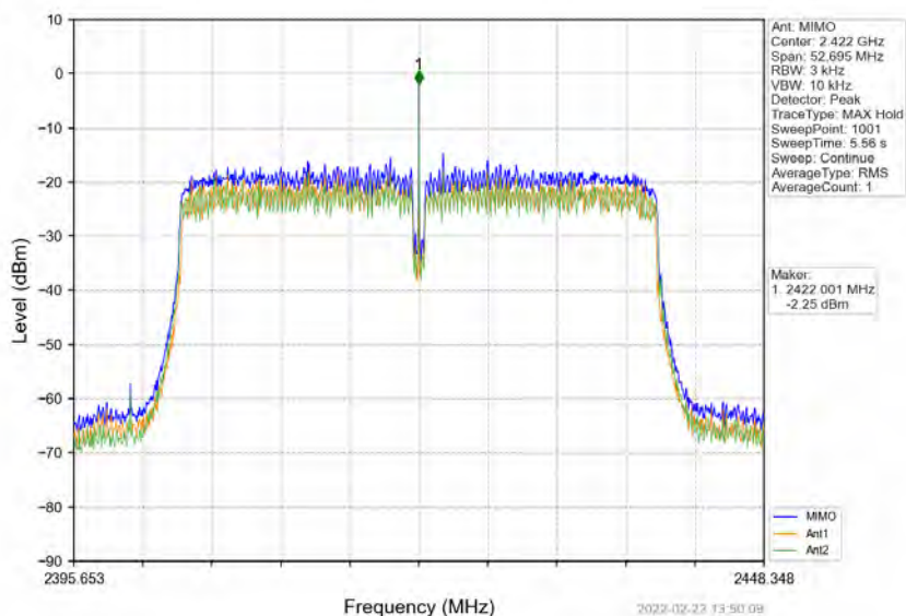
802.11n(HT40)_LCH_2422MHz_MIMO_NTNV
