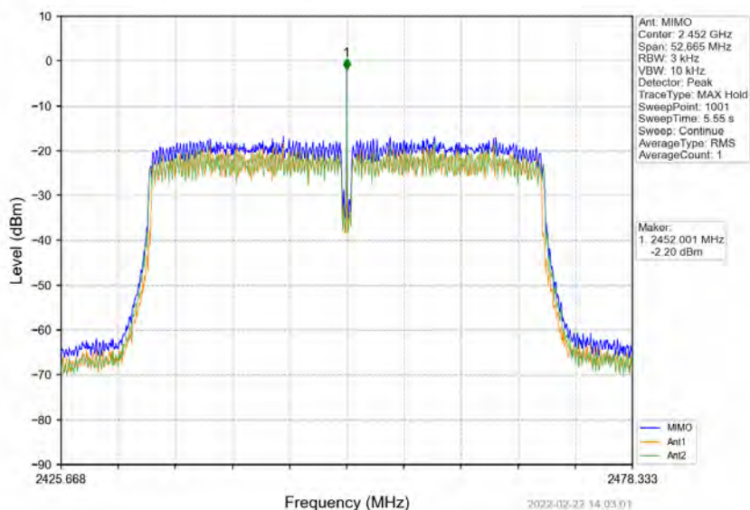
802.11n(HT40)_HCH_2452MHz_MIMO_NTNV
