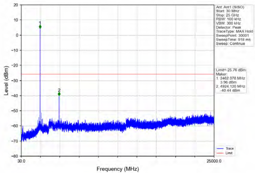
802.11b_HCH_2462MHz_Ant1 (SISO)_NTNV
