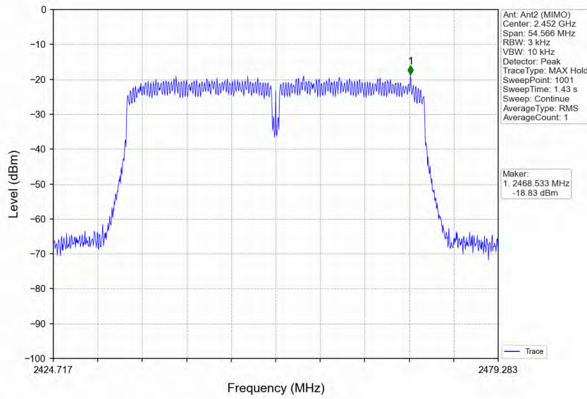
802.11n(HT40)_HCH_2452MHz_MIMO_NTNV
