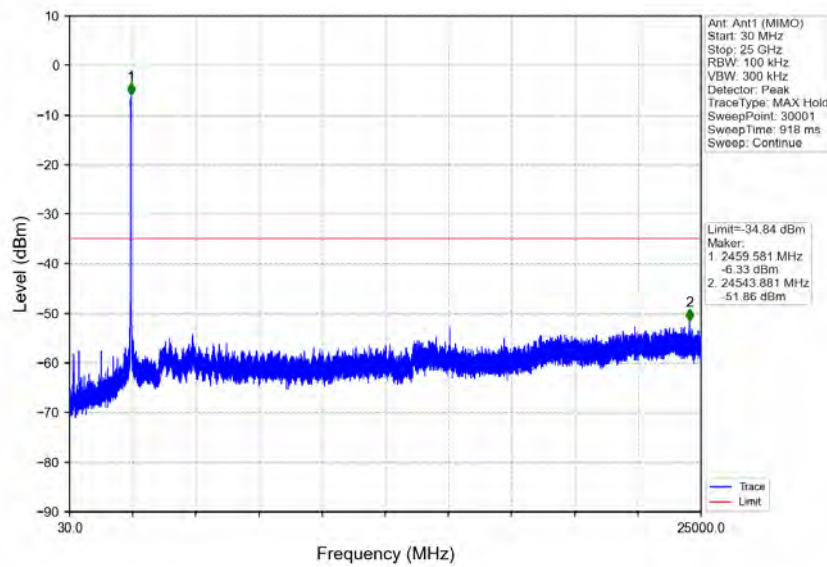
802.11n(HT40)_HCH_2452MHz_Ant1 (MIMO)_NTNV
