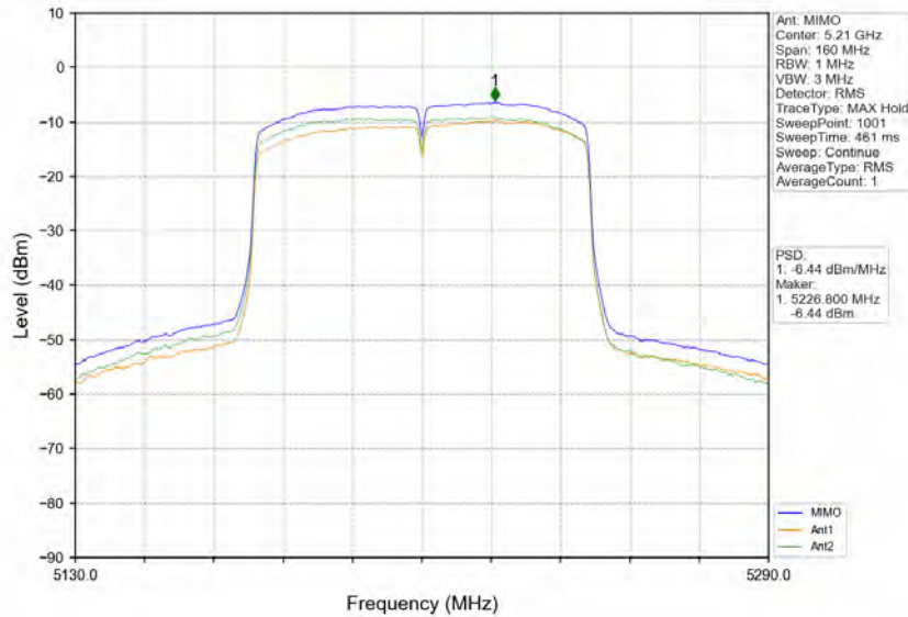
802.11ac(VHT80)_MCH_5210MHz_MIMO_NTNV
