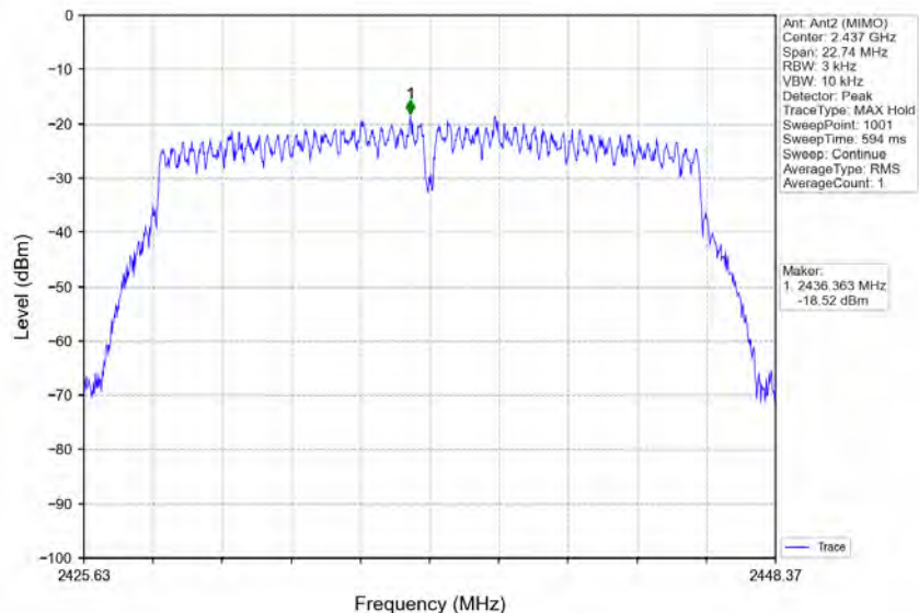
802.11n(HT20)_MCH_2437MHz_MIMO_NTNV
