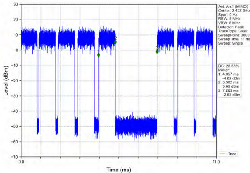
802.11n(HT40)_HCH_2452MHz_Ant1 (MIMO)_NTNV
