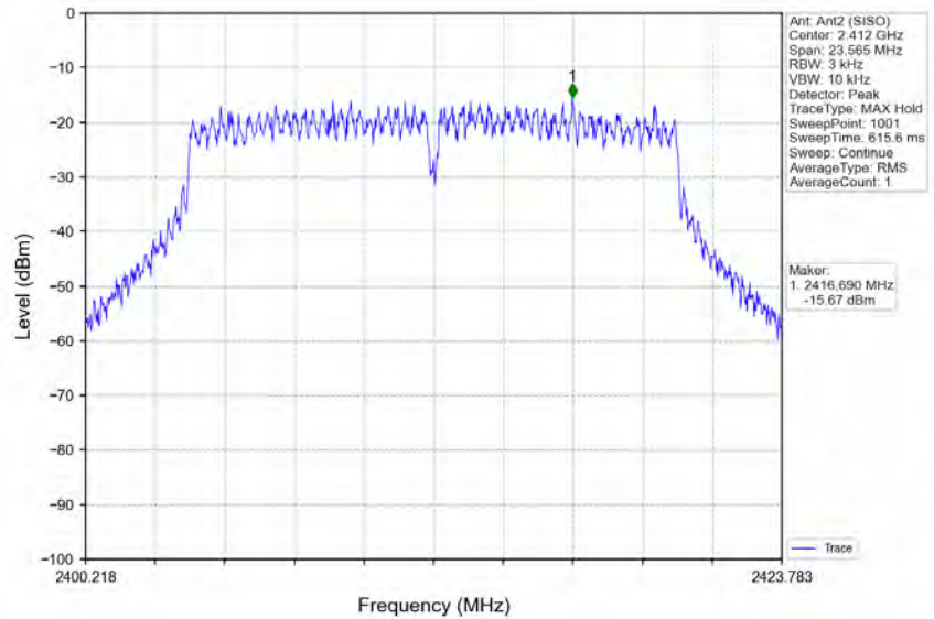
802.11g_LCH_2412MHz_Ant2 (SISO)_NTNV
