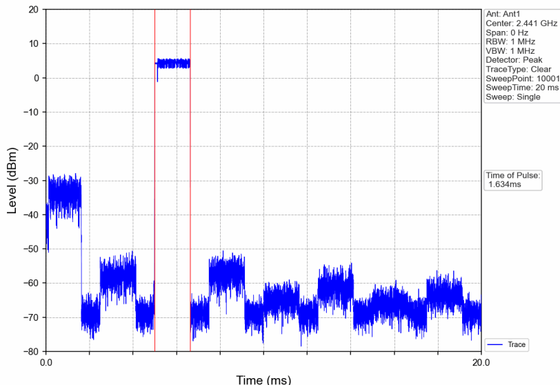
Pi/4DQPSK_2DH3_HOPP_Ant1_NTNV
