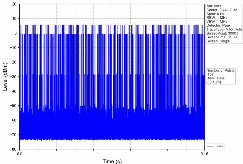
Pi/4DQPSK_2DH1_HOPP_Ant1_NTNV
