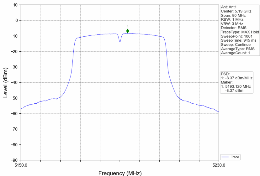
802.11n(HT40)_LCH_5190MHz_Ant1_NTNV
