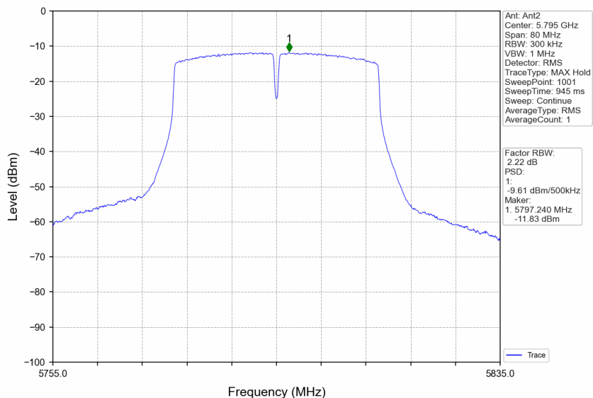
802.11n(HT40)_HCH_5795MHz_Ant2_NTNV
