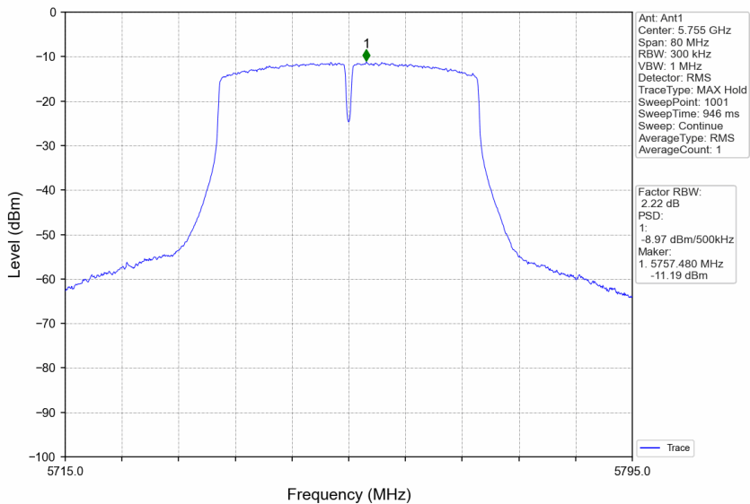
802.11n(HT40)_LCH_5755MHz_Ant1_NTNV
