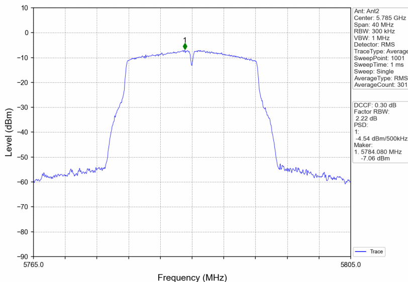
802.11a_MCH_5785MHz_Ant2_NTNV
