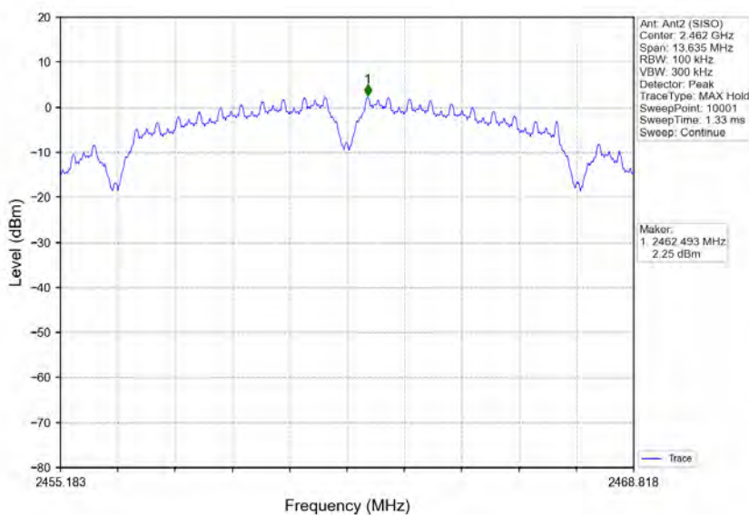
802.11b_HCH_2462MHz_Ant2 (SISO)_NTNV
