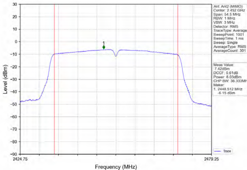
802.11n(HT40)_HCH_2452MHz_Ant2 (MIMO)_NTNV
