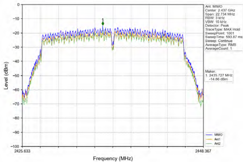
802.11n(HT20)_MCH_2437MHz_MIMO_NTNV
