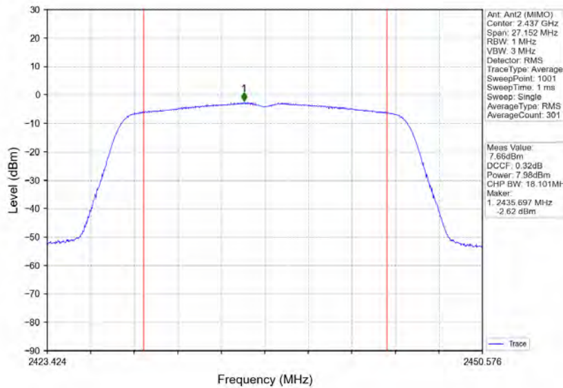
802.11n(HT20)_MCH_2437MHz_Ant2 (MIMO)_NTNV
