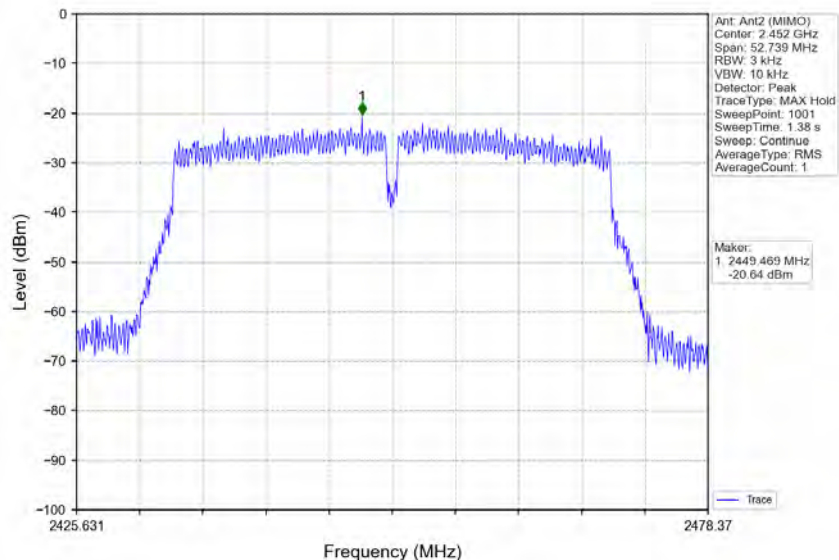
802.11n(HT40)_HCH_2452MHz_MIMO_NTNV
