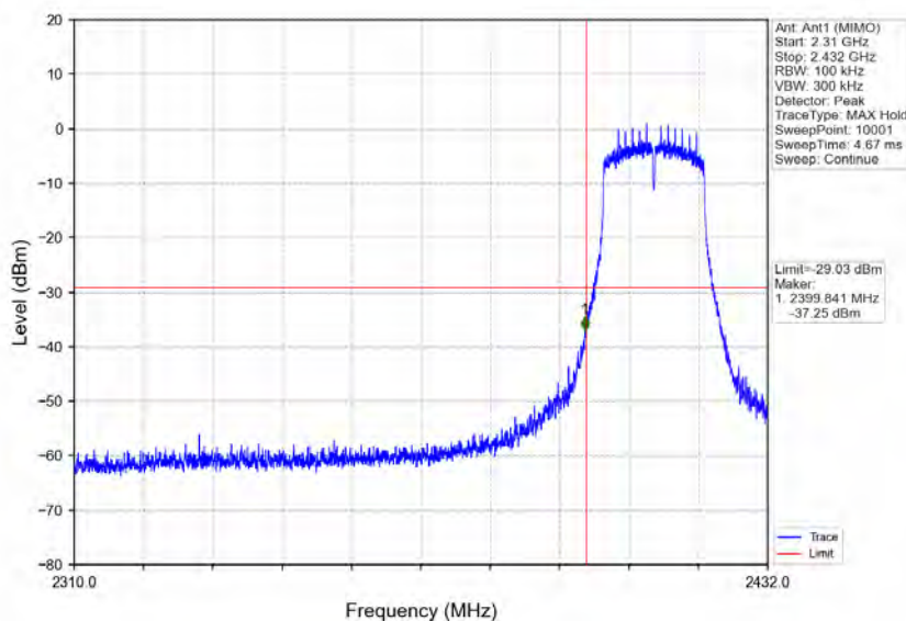
802.11n(HT20)_LCH_2412MHz_Ant1 (MIMO)_NTNV
