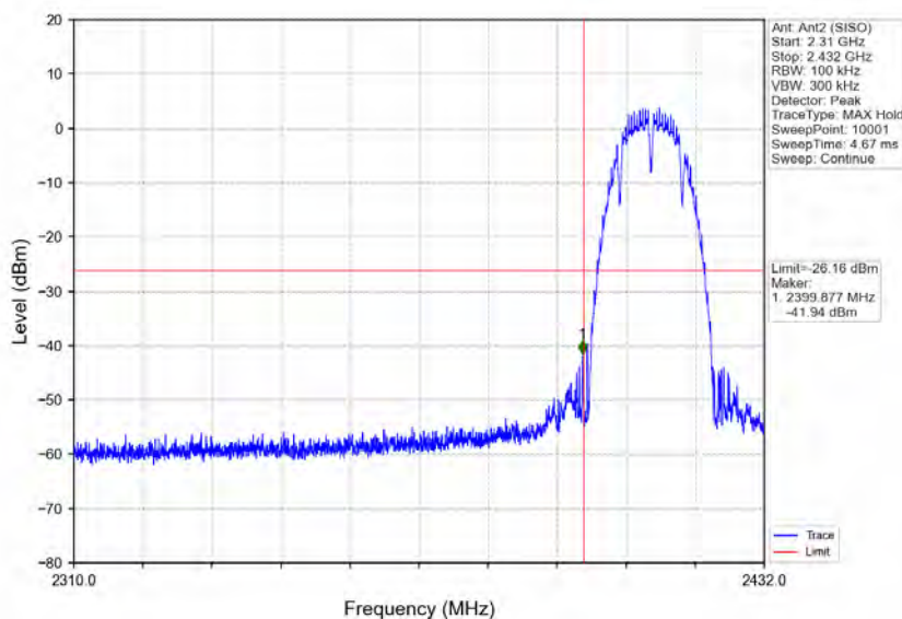
802.11b_LCH_2412MHz_Ant2 (SISO)_NTNV
