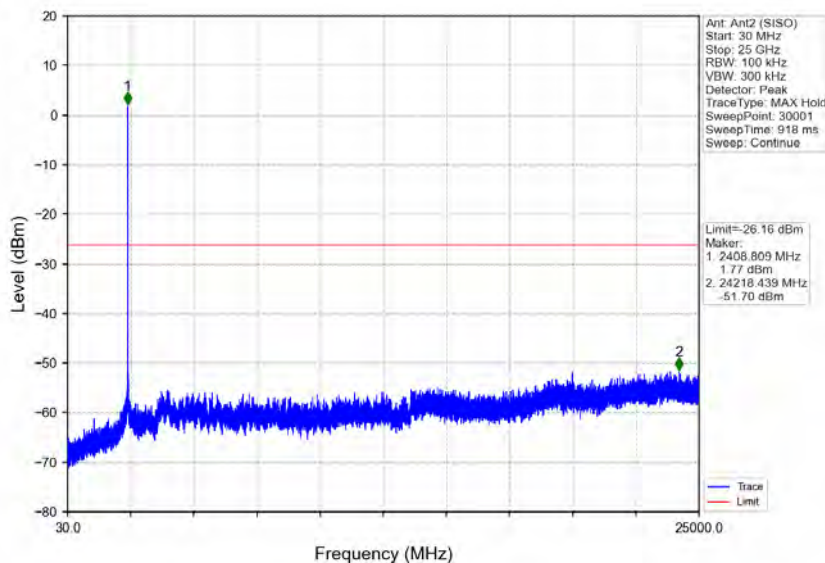
802.11b_LCH_2412MHz_Ant2 (SISO)_NTNV
