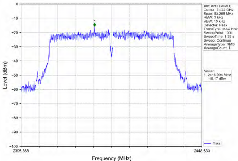
802.11n(HT40)_LCH_2422MHz_MIMO_NTNV
