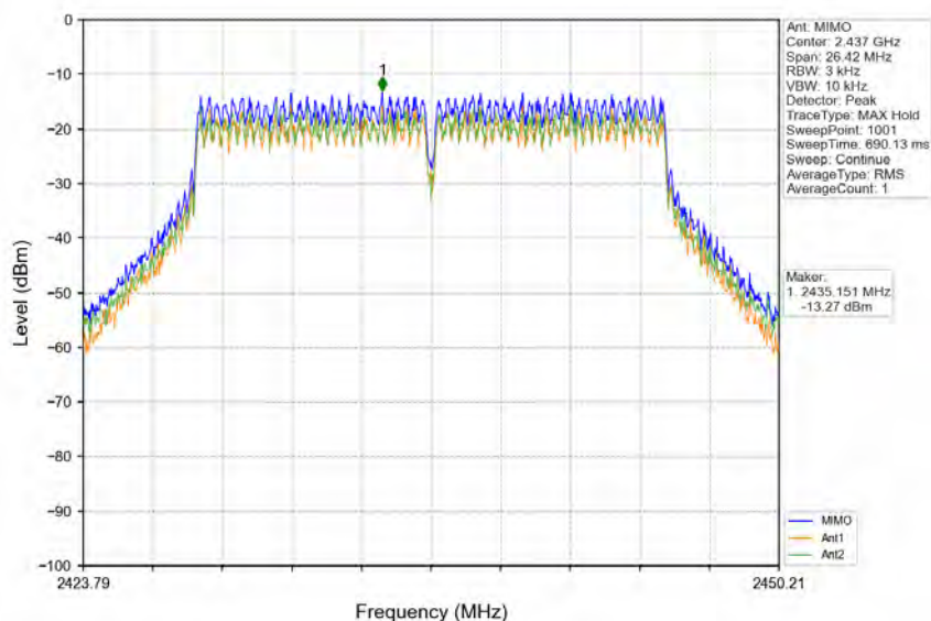
802.11n(HT20)_MCH_2437MHz_MIMO_NTNV
