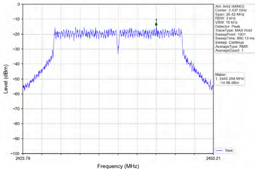
802.11n(HT20)_MCH_2437MHz_MIMO_NTNV
