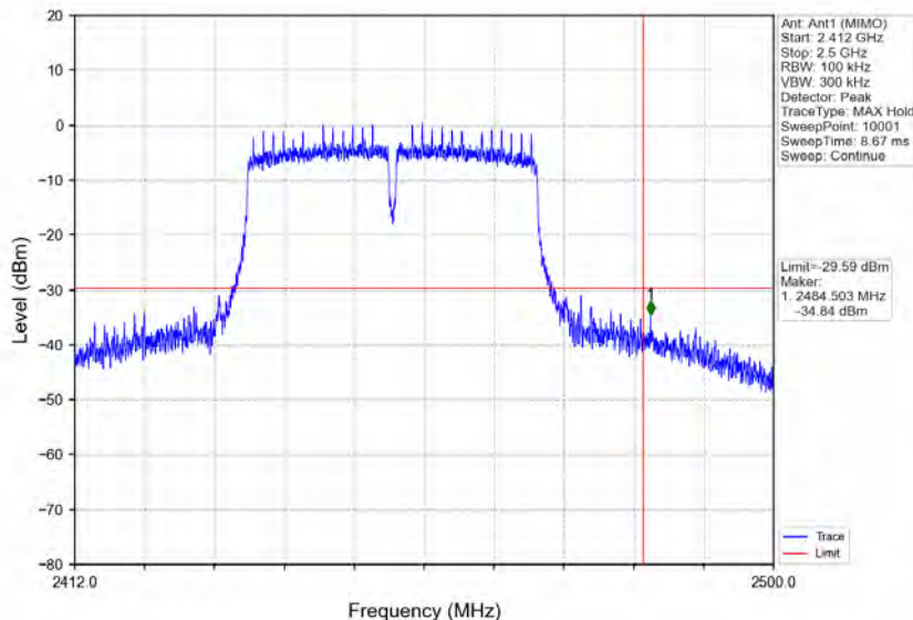
802.11n(HT40)_HCH_2452MHz_Ant1 (MIMO)_NTNV
