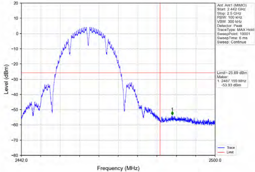
802.11n(HT20)_HCH_2462MHz_Ant1 (MIMO)_NTNV
